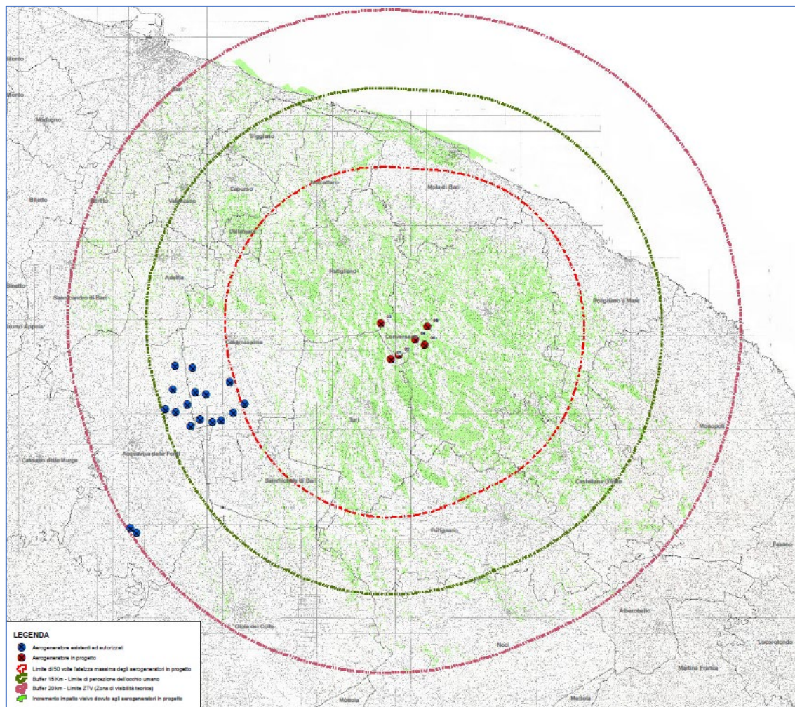
Figura 8 -Inquadramento del Parco eolico rispetto agli altri aerogeneratori esistenti
