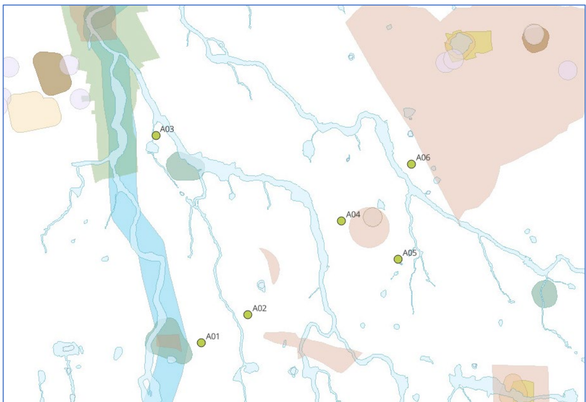
Figura 3 - Ipotesi Layout a 6 aerogeneratori con collocazione differente - analisi aree non idonee FER
