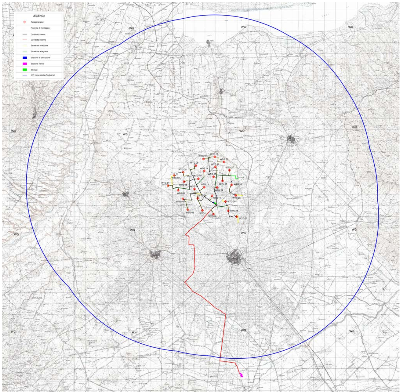
Inquadramento su IGM, scala 1:50.000
