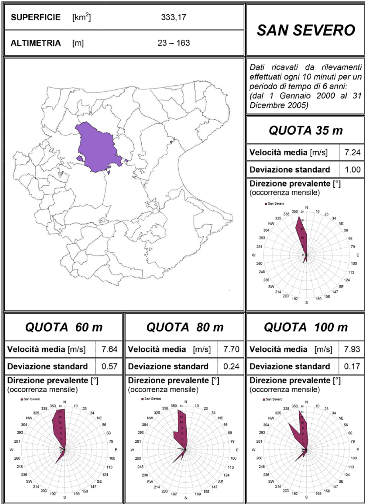
Figura 1 Ventosità alle quote di 35-60-80-100 nel comune di San Severo (FG)-Università degli studi di Lecce-Progetto M.E.T.E.
