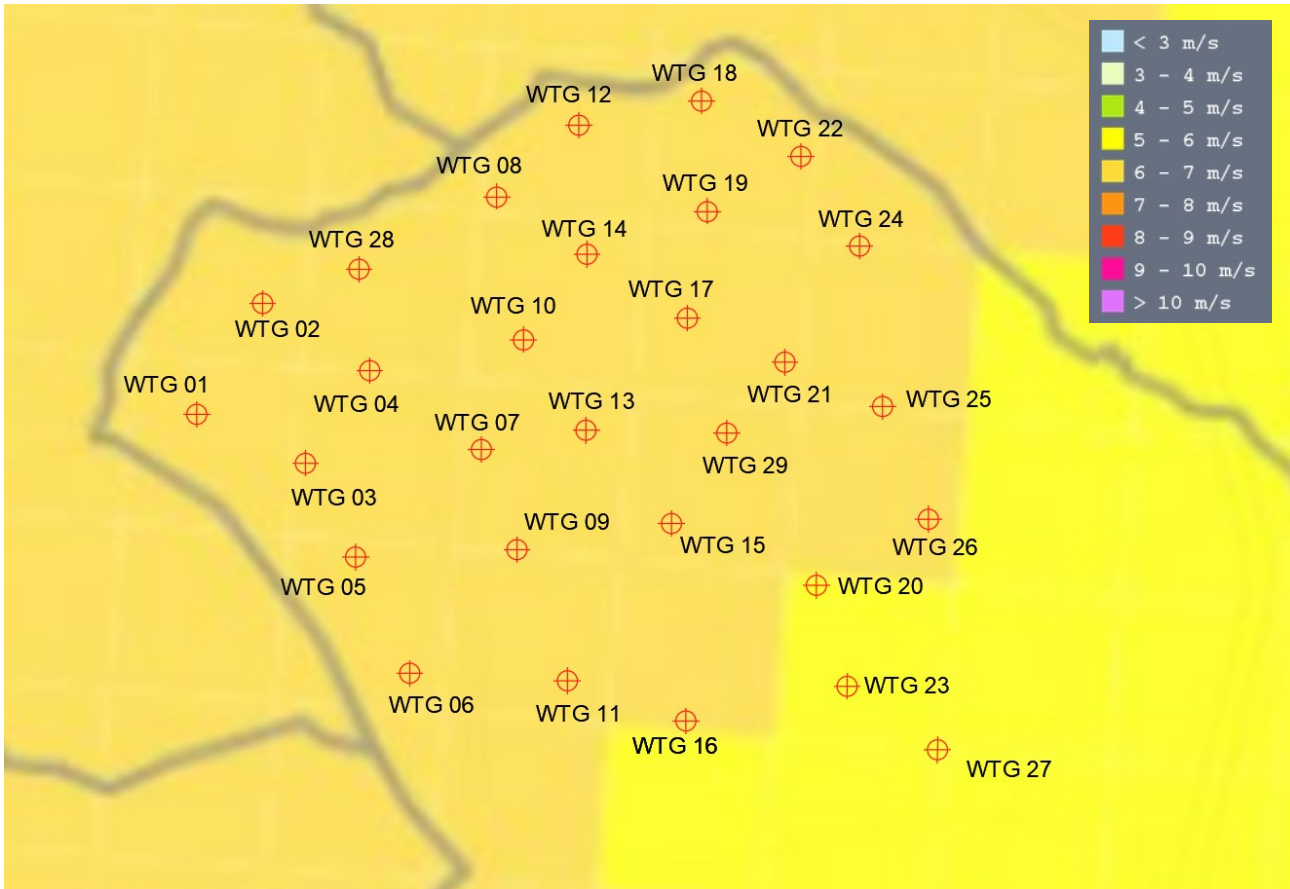
Impianto su Atlante eolico interattivo con velocità media annua del vento a 150 m s.l.m.
