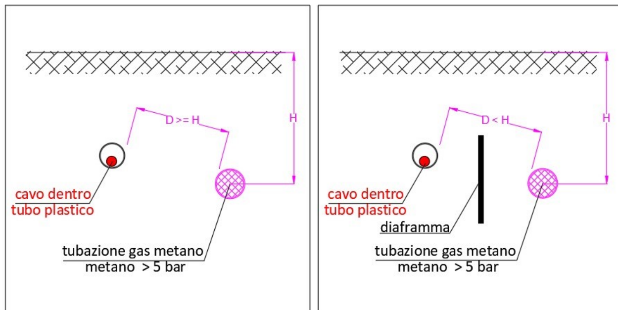
Figura 10 Parallelismi cavidotto energia e tubazioni o serbatoi con pressione > 5 bar
