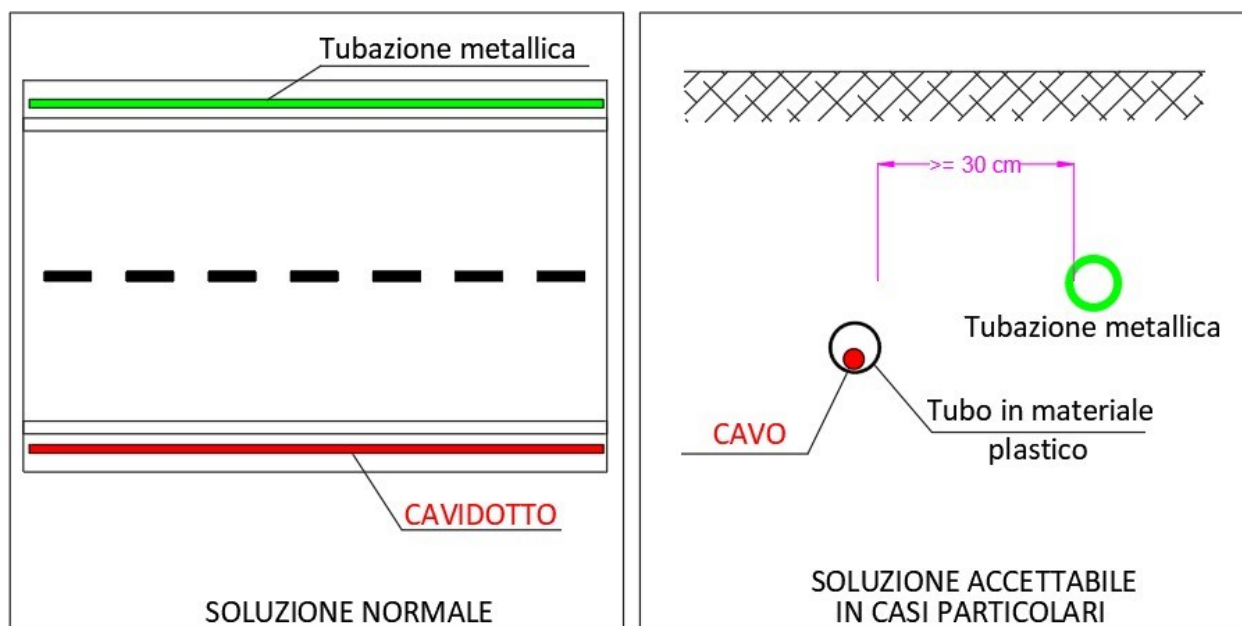
Figura 6 Parallelismi fra cavi di energia e tubazioni metalliche
