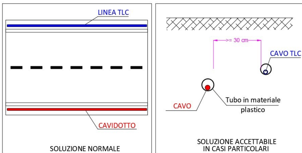
Figura 4 Parallelismo tra cavi energia e linee di telecomunicazione
