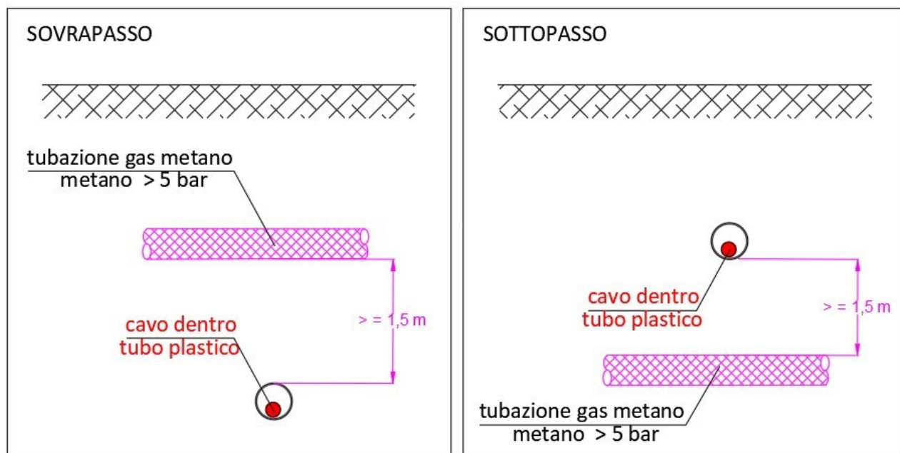
Figura 8 Coesistenza tra cavidotti energia e tubazioni o serbatoi del gas metano
