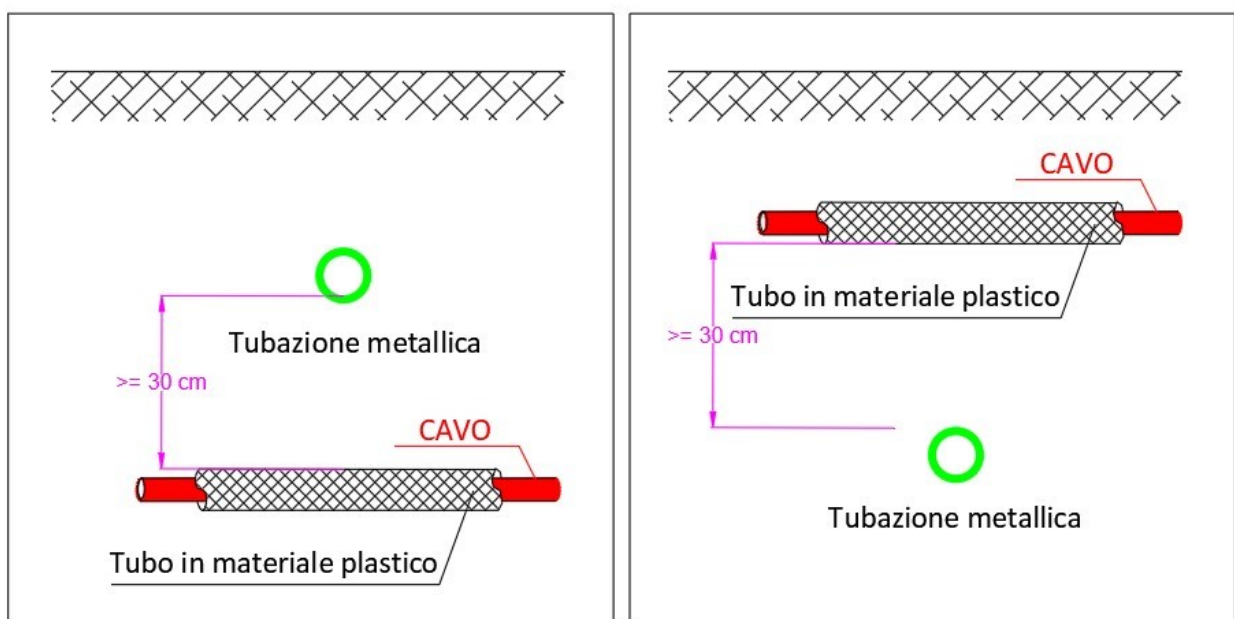
Figura 5 Incroci fra cavi di energia e tubazioni metalliche
