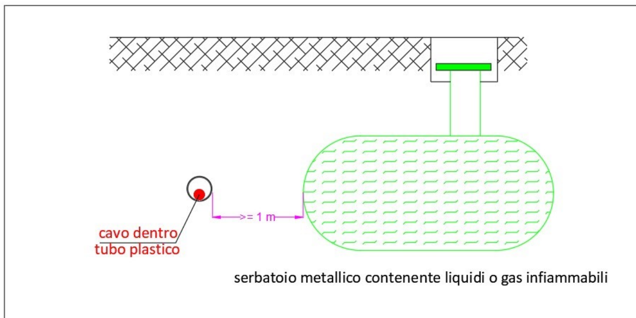
Figura 7 Coesistenza tra cavi energia e serbatoi di liquidi/gas infiammabili
