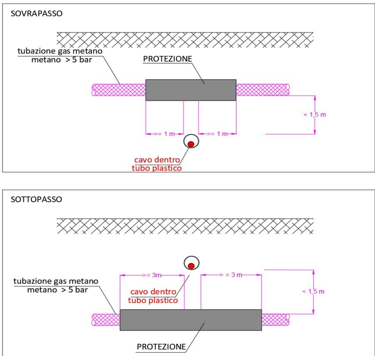
Figura 9 Incrocio cavidotto energia e tubazioni o serbatoi gas metano con pressione >5 bar
