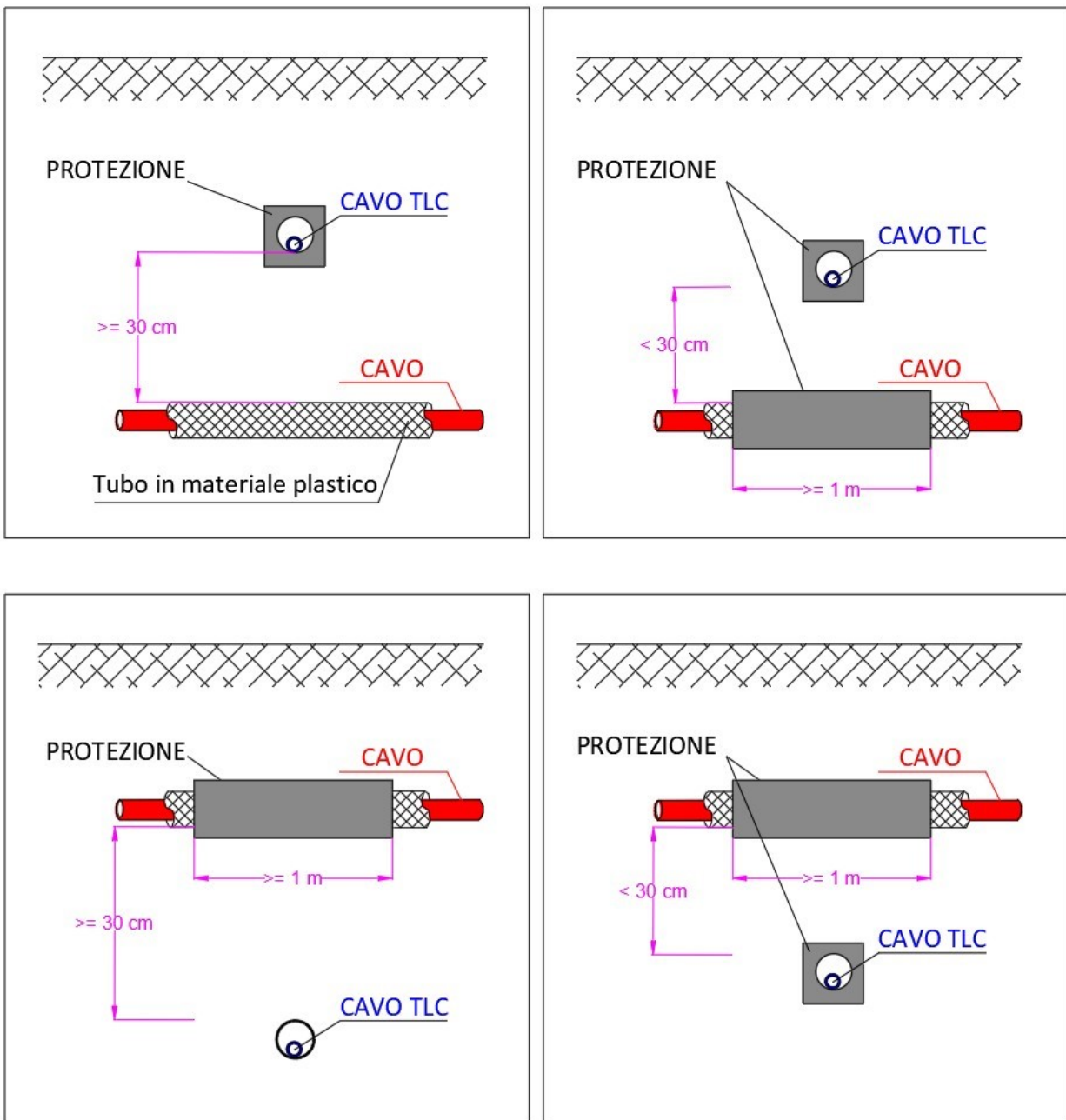
Figura 3 Incrocio tra cavi energia e linee di telecomunicazione
