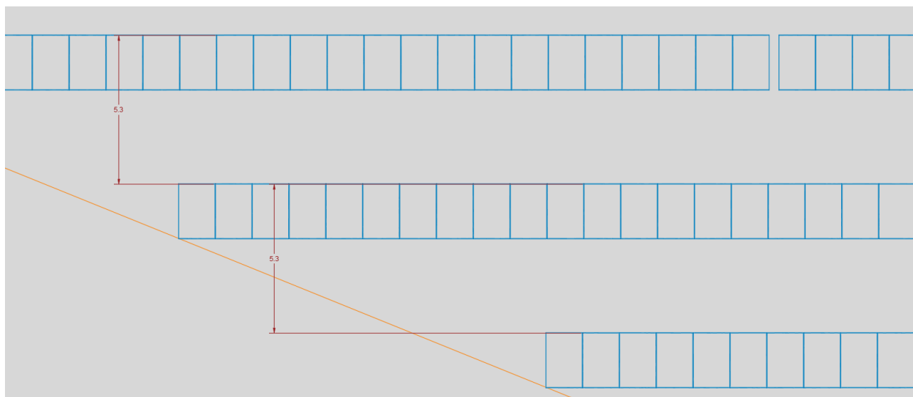
Figura 3-3 Distanza interfila - Impianto di Riferimento
