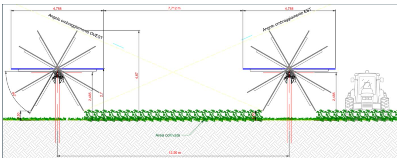
Figura 3.1 – Tipico struttura di sostegno
