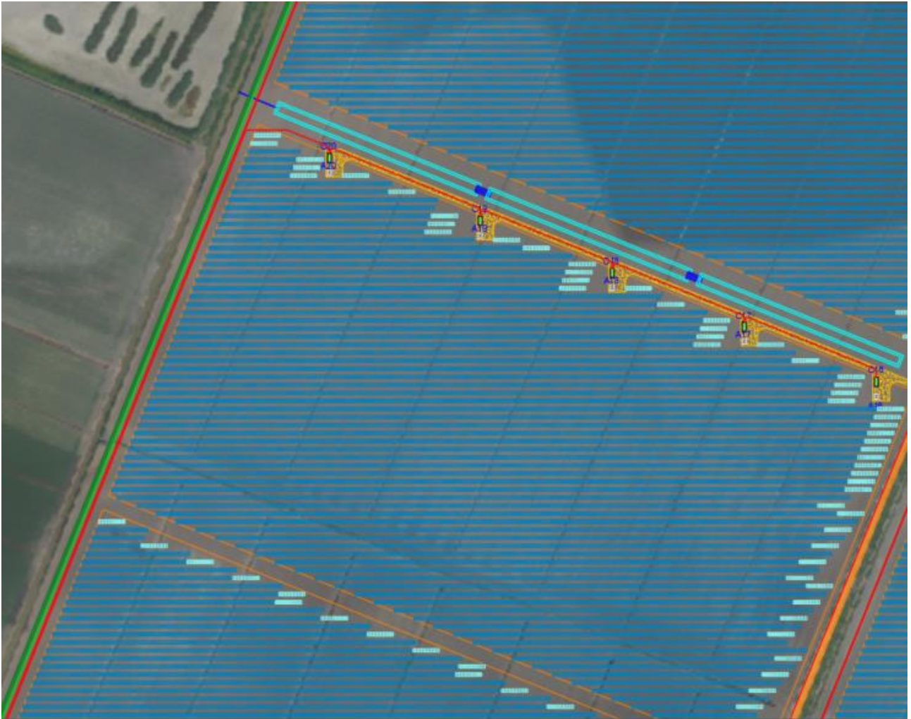
Figura 3-2 Inquadramento sottocampo - Impianto di Riferimento
