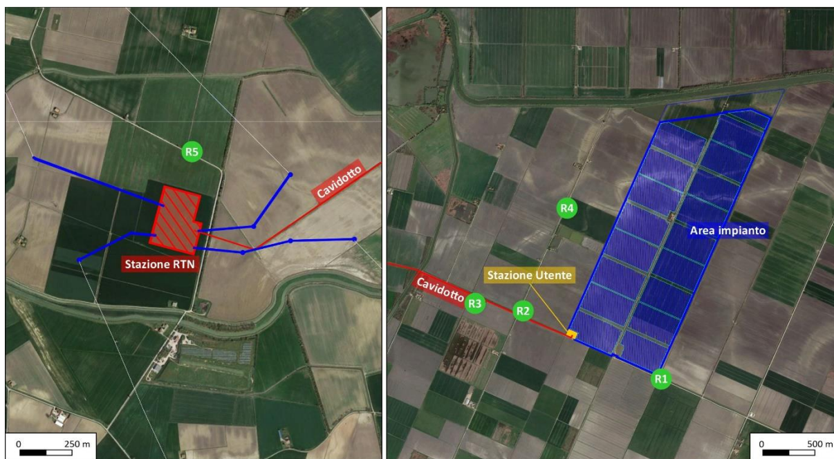
Figura 4 – Recettori più prossimi individuati nei pressi dell’impianto agrivoltaico e delle opere di Rete
