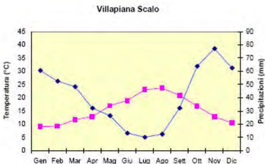
Figura. 1. Diagramma ombro-termico di Bagnouls e Gaussen
