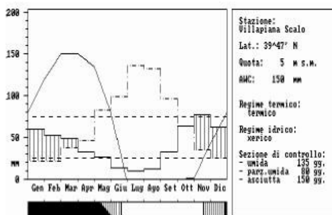
Figura 2. Elaborazione dati di umidità
