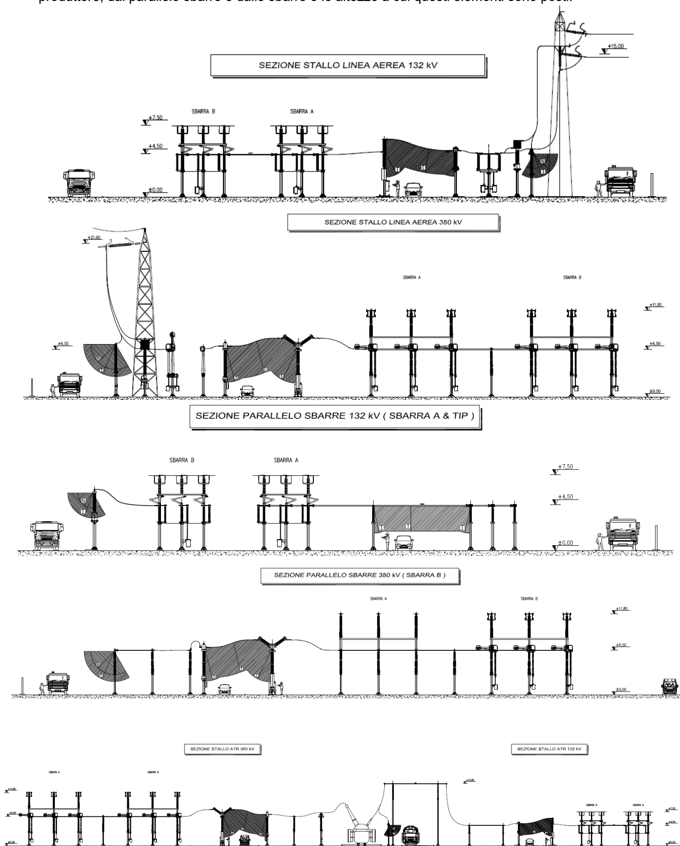
Figura 4 – Sezioni degli stalli linea e delle sbarre delle due sezioni 380 e 132 kV di una stazione standard Terna
