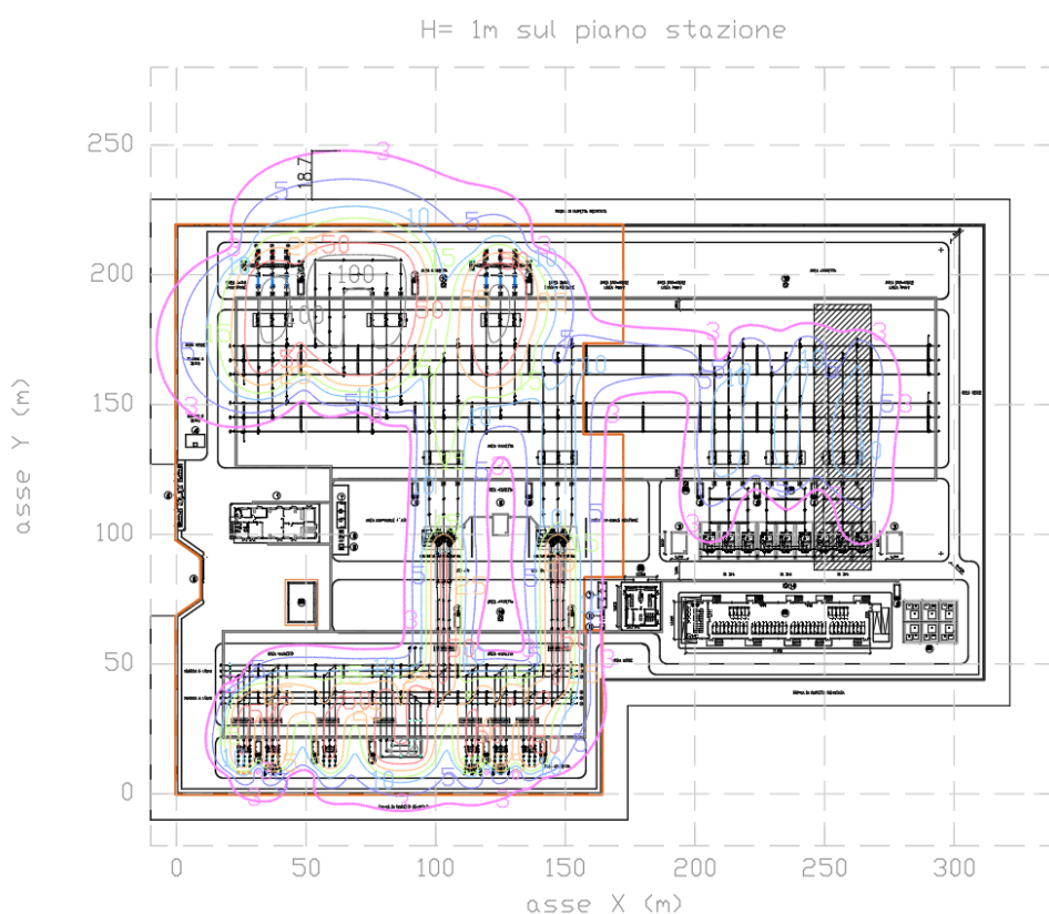
Figura 7 – Livelli di campo magnetico a 1 m dal piano della stazione
