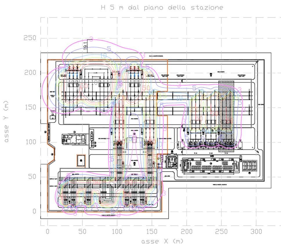
Figura 8 – Livelli di campo magnetico a 5 m dal piano della stazione
