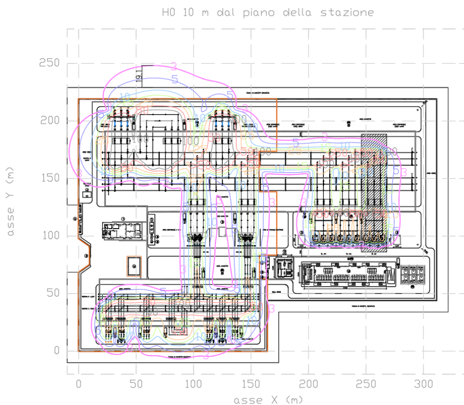
Figura 9 – Livelli di campo magnetico a 10 m dal piano della stazione
