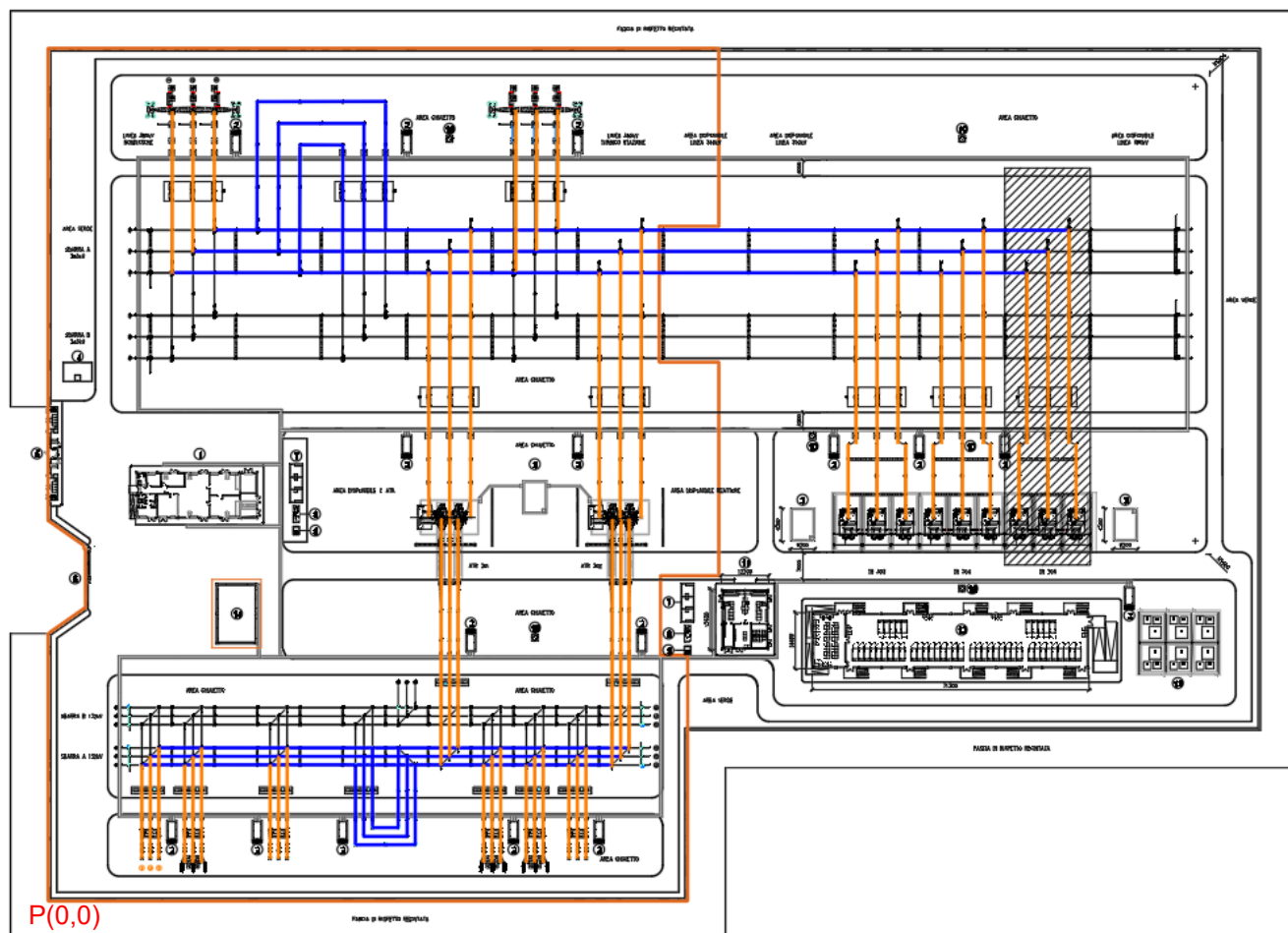
Figura 5 – Schematizzazione degli elementi attivi all'interno della planimetria
