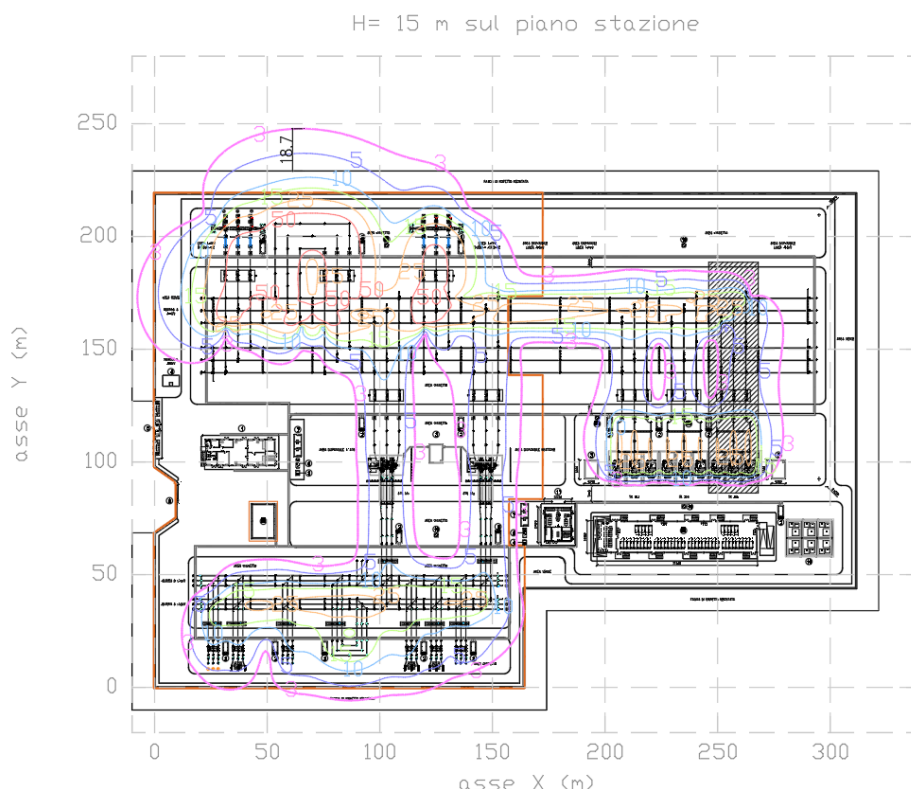
Figura 10 – Livelli di campo magnetico a 15 m dal piano della stazione
