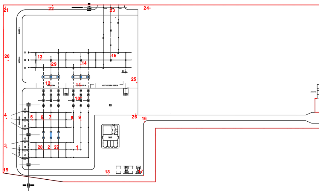
Figura 3 – Planimetria della stazione 380 kV Voghera esistente
