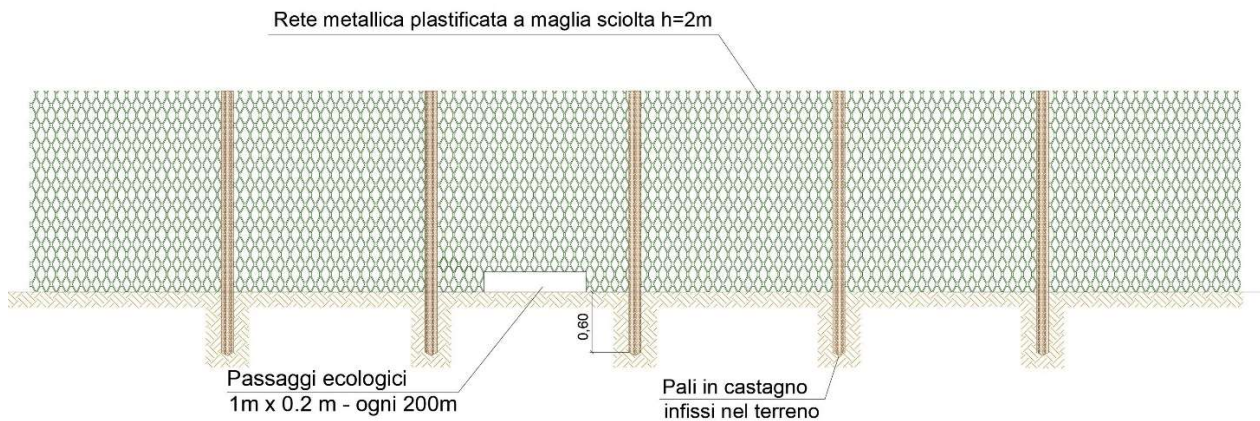
Figura 3 – Recinzione perimetrale
