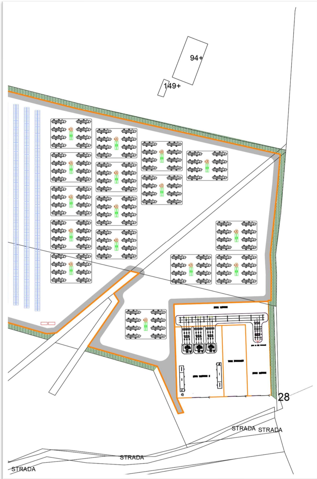
Figura 1 - Layout Impianto Storage BEES
