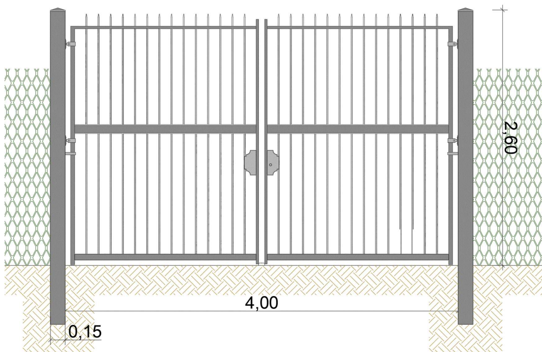
Figura 2 - Cancello d'ingresso
