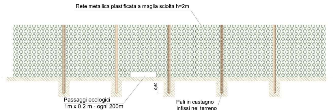
Figura 1 - Prospetto recinzione
