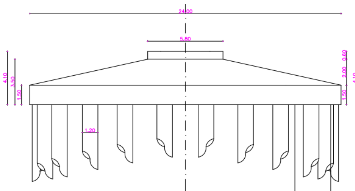
Figura 13 - Tipologia fondazione (sezione)
