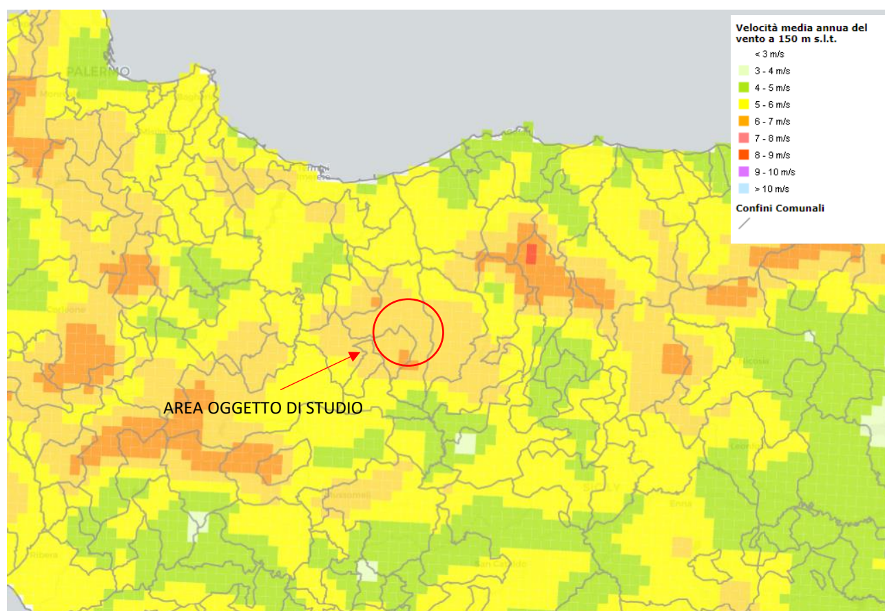
Figura 9 - Velocità media annua del vento a 150 m s.l.t. (fonte: Atlante Eolico Nazionale)
