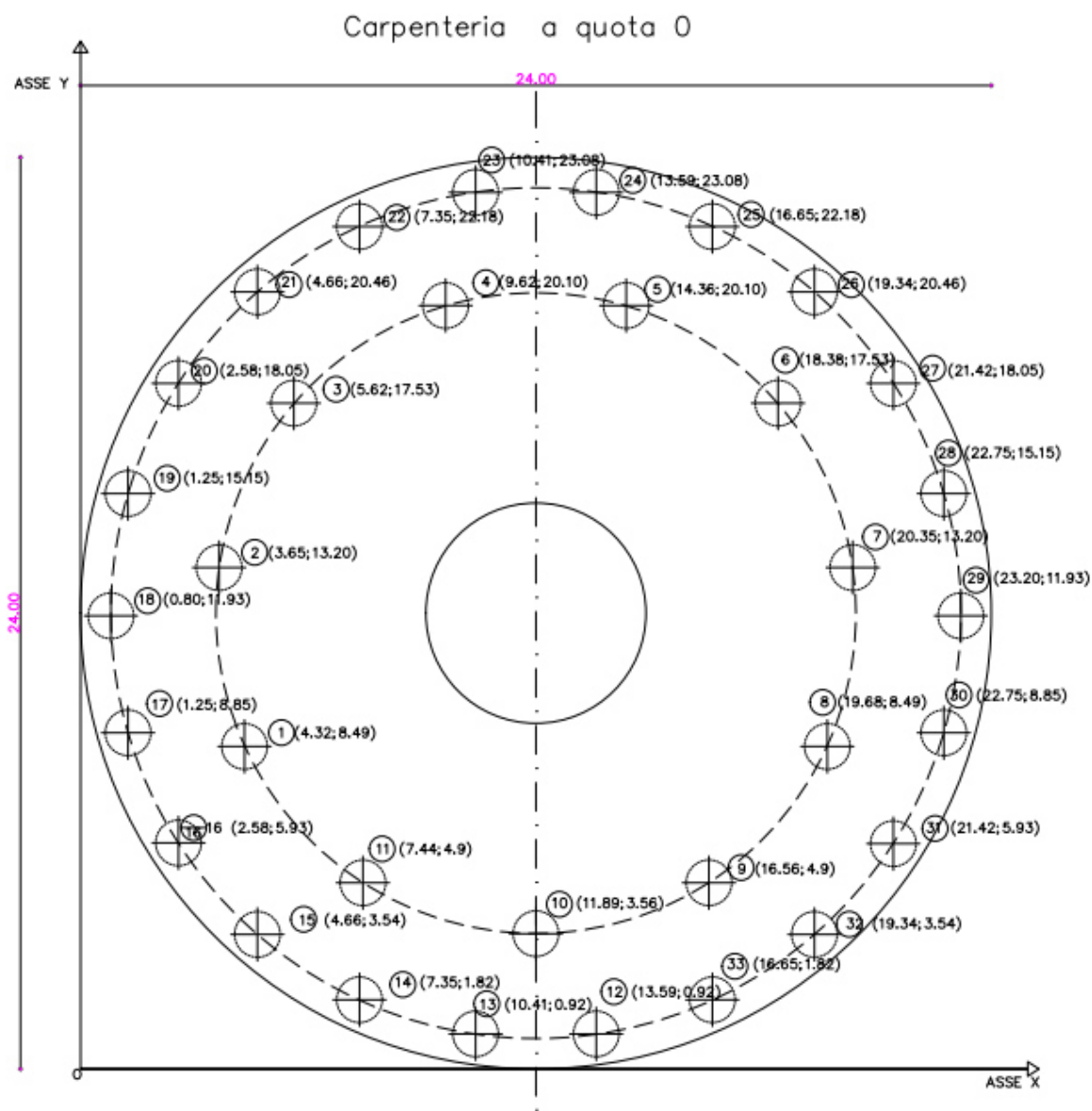
Figura 12 - Tipologia fondazione (pianta)
