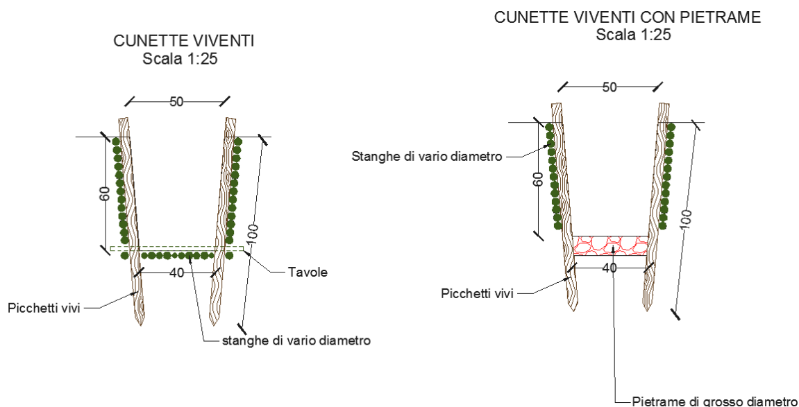
Figura 24 – Sezioni tipo di cunette viventi
