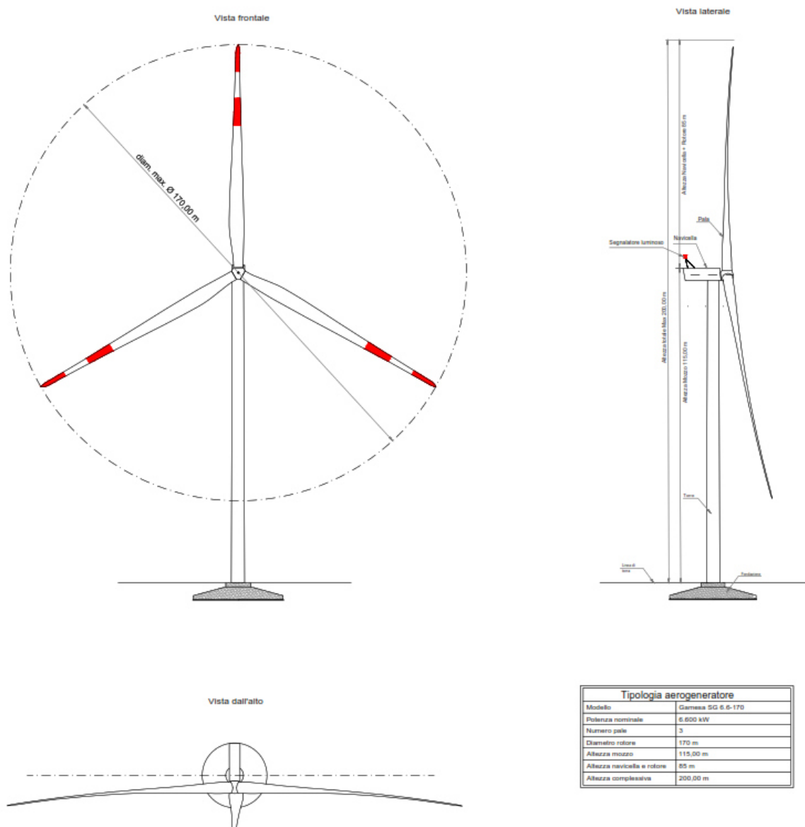
Figura 31 - Pianta e prospetti aerogeneratore
