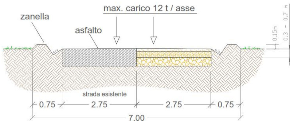
Figura 19 - Adeguamento della carreggiata in presenza di carreggiata esistente in asfalto
