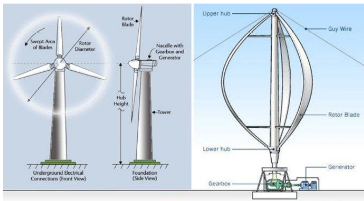
Figura 32 - Schema tipo di turbine ad asse orizzontale e verticale
