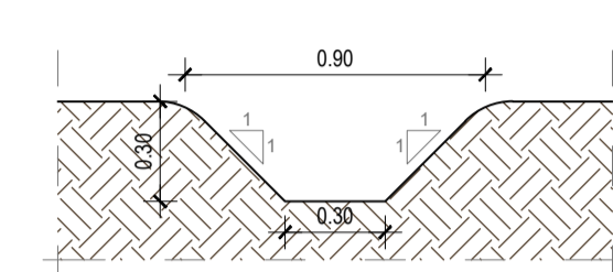
PARTICOLARE FOSSO DI GUARDIA scala 1:25
