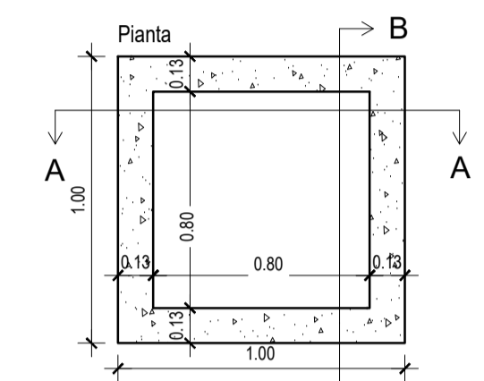
PARTICOLARE POZZETTO E CHIUSINO scala 1:25
