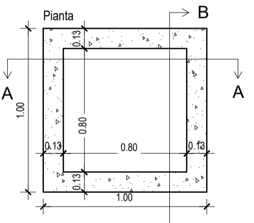
PARTICOLARE POZZETTO E CHIUSINO scala 1:25
