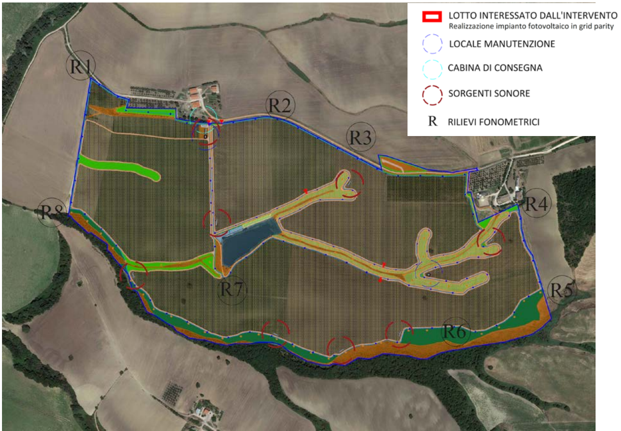
Figura 4: Individuazione punti di misura e sorgenti sonore – Area Progetto Morrone
