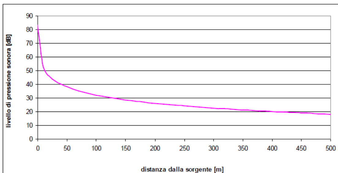
Figura 114: Curva di abbattimento sonora – propagazione diretta
