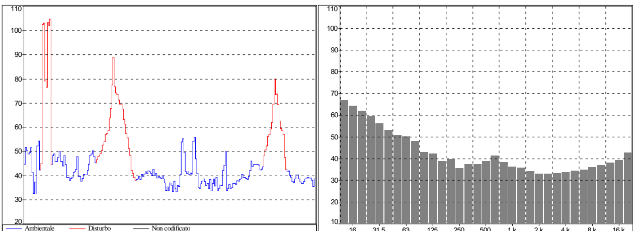
Figura 11: Dettaglio rilievo R6 – Area Progetto Morrone
