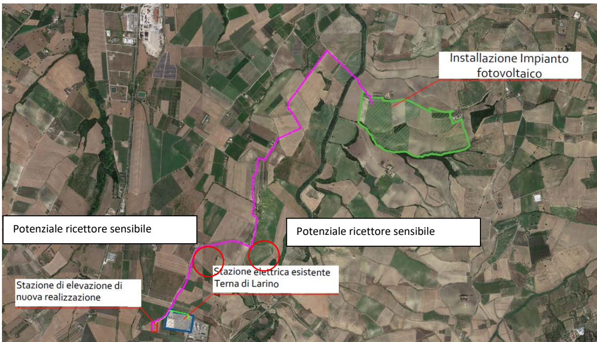
Figura 5: Inquadramento territoriale – Area Progetto cavidotto "Morrone"
