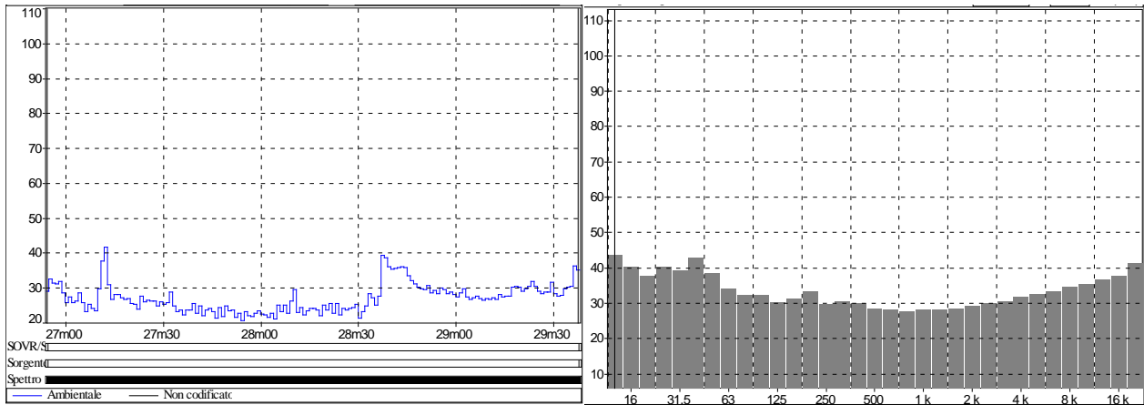
Figura 12: Dettaglio rilievo R7 – Area Progetto Morrone
