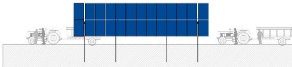
Figura 3-4: Vista frontale della struttura di supporto dei moduli.
