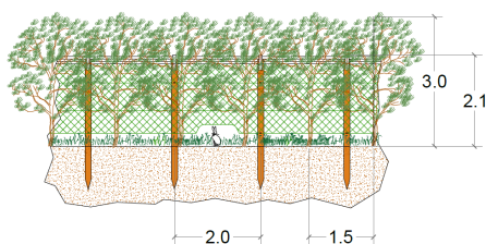
Figura 3-5: Recinzione e mitigazione fascia alberata perimetrale.
