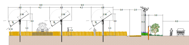
Figura 3-3: Vista in sezione delle strutture di supporto dei moduli con quotatura.
