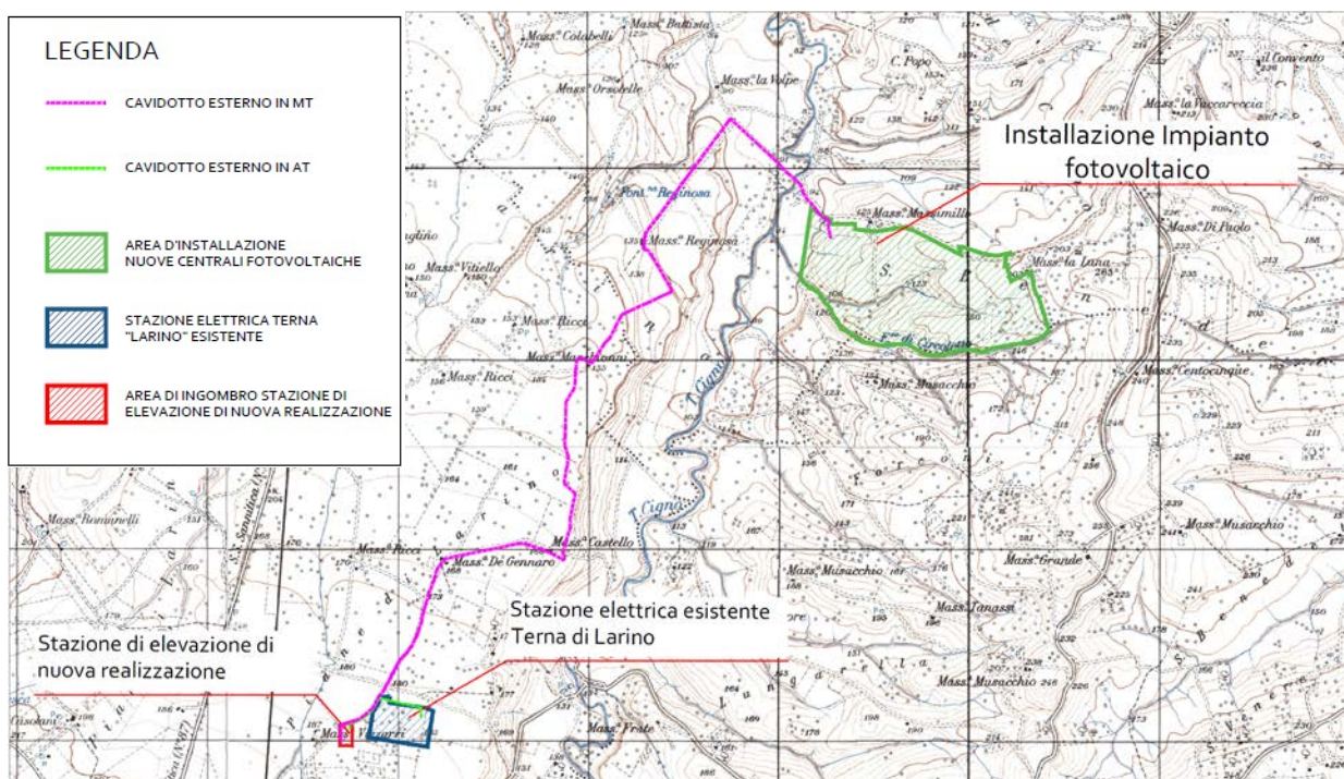
Figura 2 - Impianto agrovoltaico e Stazione elettrica Terna + cavidotti interrati MT/AT su base IGM
