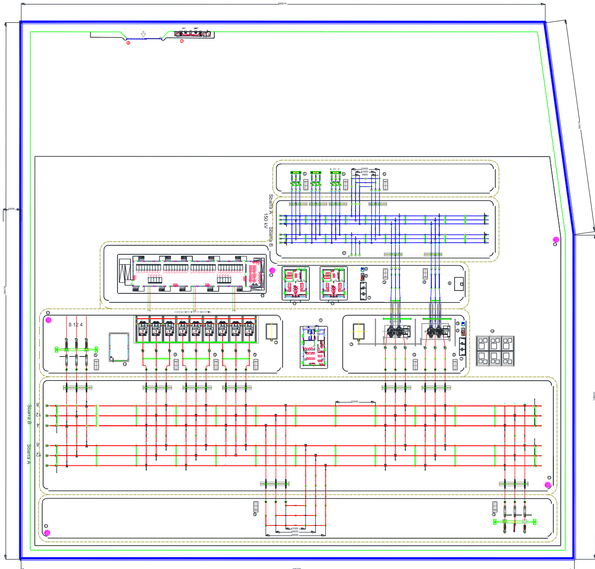
Figura 7 - PLANIMETRIA ELETTROMECCANICA GENERALE
