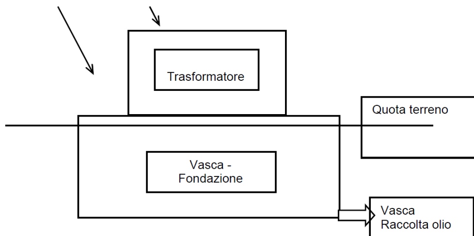
Figura 10 - SCHEMA DELLA FUNZIONE VASCA FONDAZIONE
