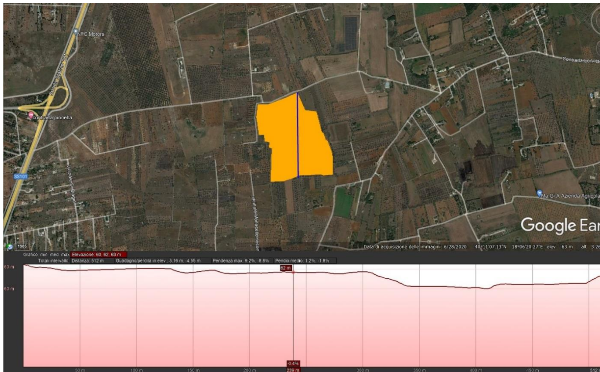
Figura 8 - PROFILO LONGITUDINALE
