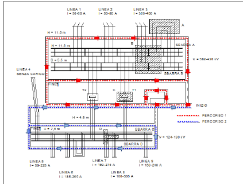
Figura 5 - PIANTA DI UNA TIPICA STAZIONE 380/132 KV CON L'INDICAZIONE DELLE PRINCIPALI DISTANZE FASE-FASE (S) E FASE-TERRA (H), E DELLE VARIAZIONI DELLE TENSIONI E DELLE CORRENTI DURANTE LE MISURAZIONI DI CAMPO ELETTRICO E MAGNETICO
