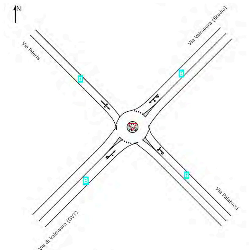
Figura 21 – Livello di Servizio per corsia – Scenario di cantiere B
