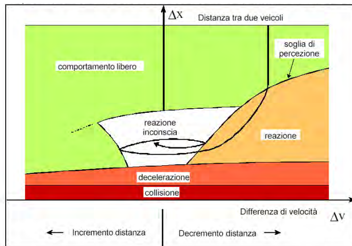
Figura 12 - Modello di successione dei veicoli secondo WIEDEMANN
