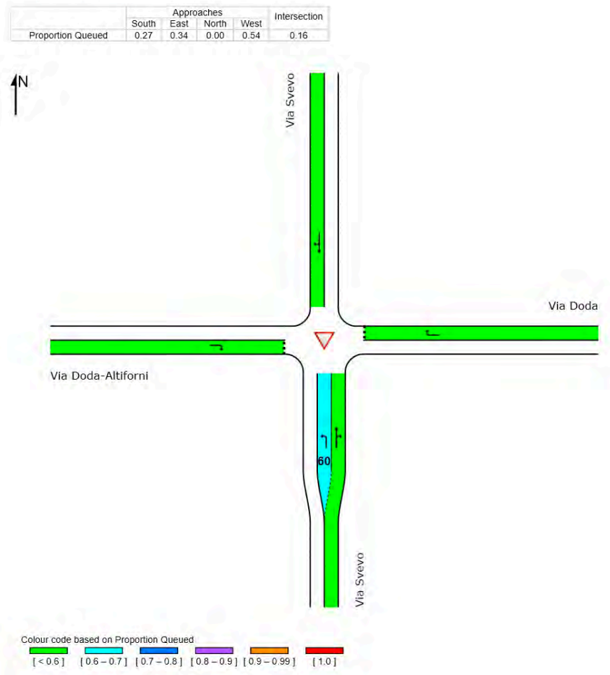
Figura 14 – Proporzione di traffico in coda – Stato attuale
