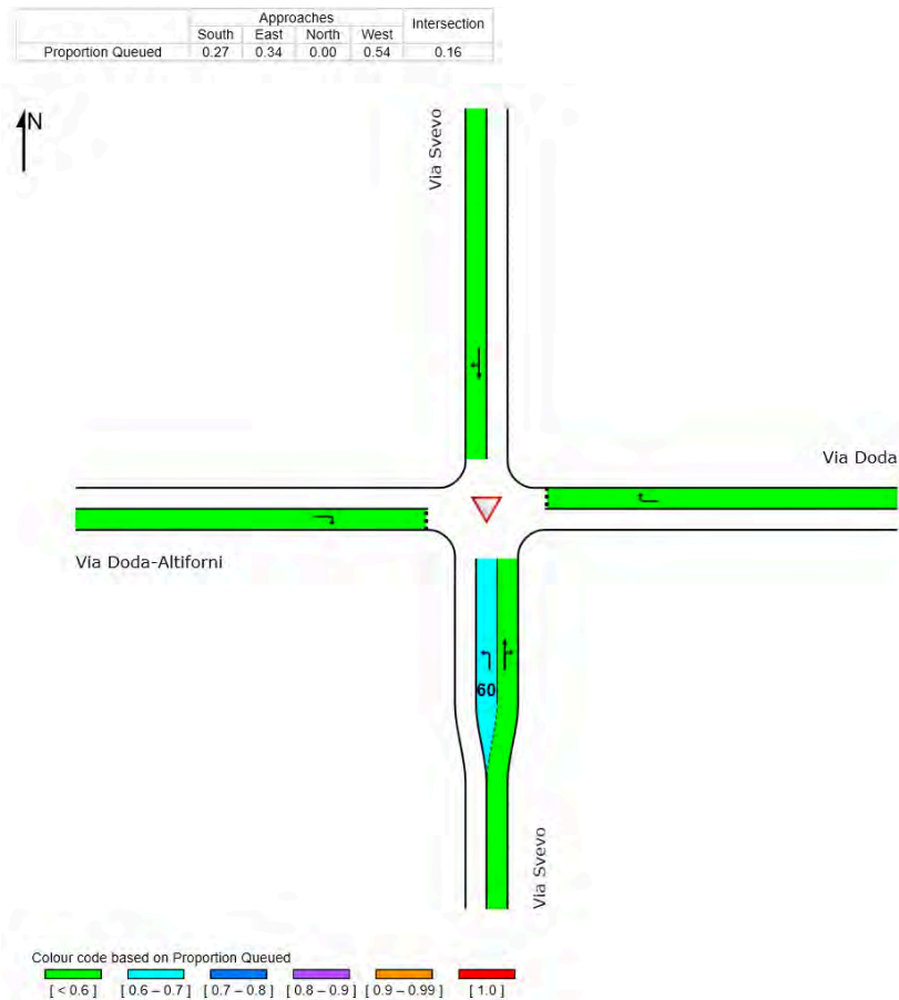
Figura 24 – Proporzione di traffico in coda – Scenario di cantiere C
