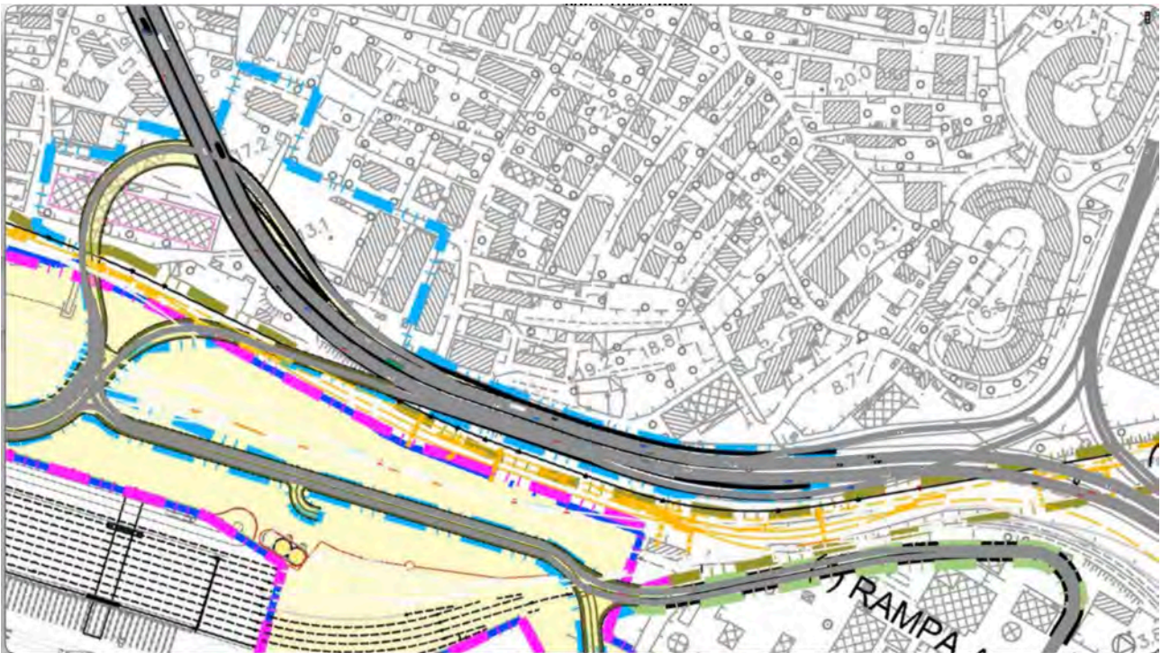
Figura 27 – Schema delle rampe nel modello di simulazione
