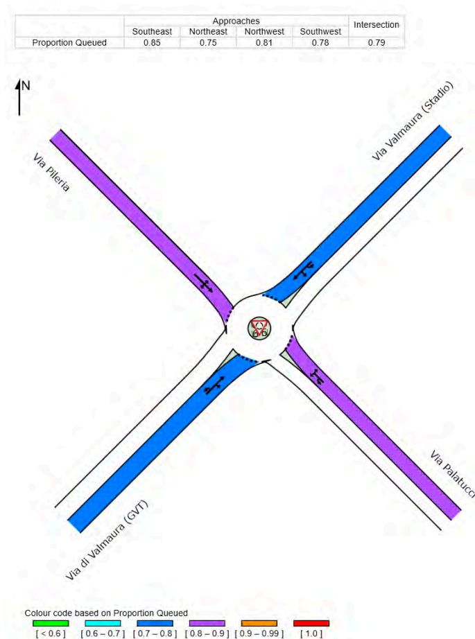
Figura 22 – Proporzione di traffico in coda – Scenario di cantiere B
