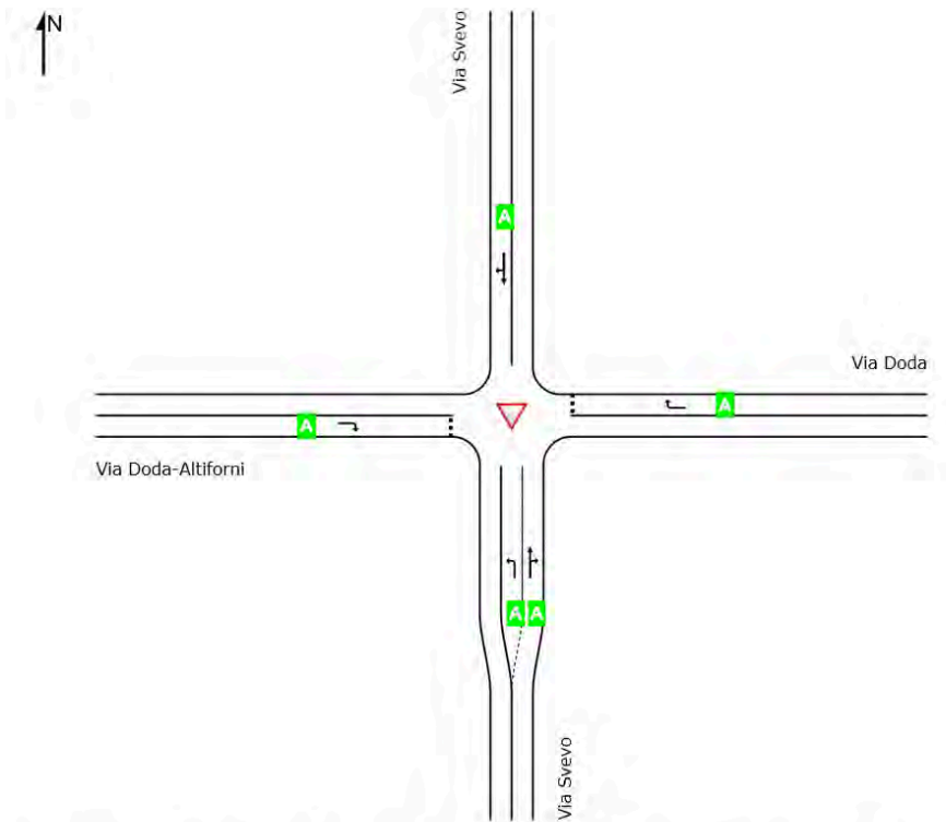
Figura 23 – Livello di Servizio per corsia – Scenario di cantiere C
