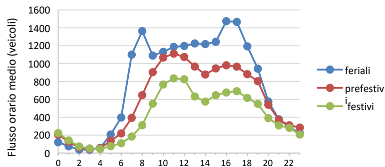
Andamento orario medio dei flussi di traffico - Direzione Ascendente
