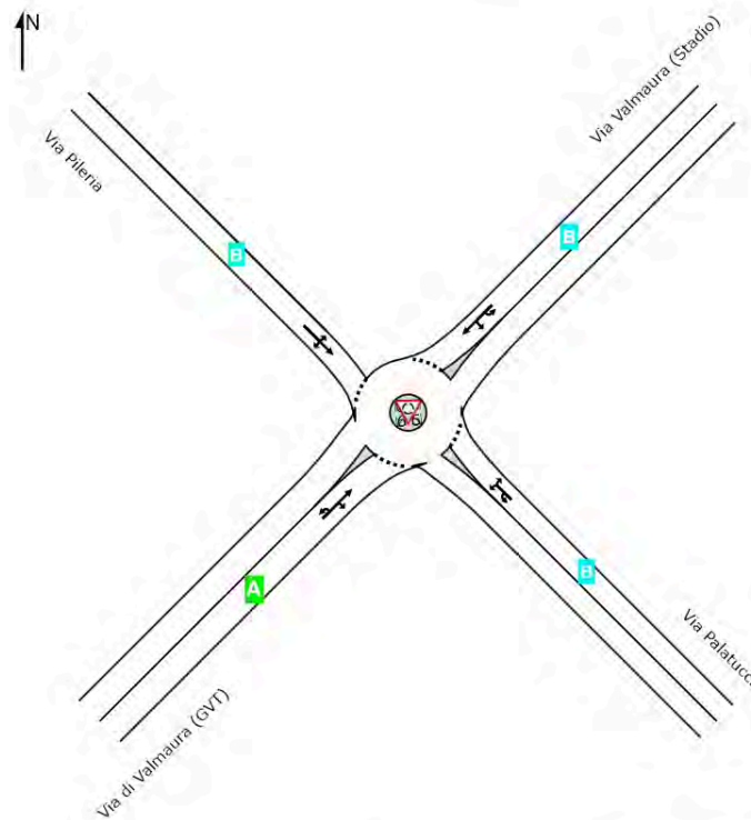
Figura 15 – Livello di Servizio per corsia – Stato attuale
