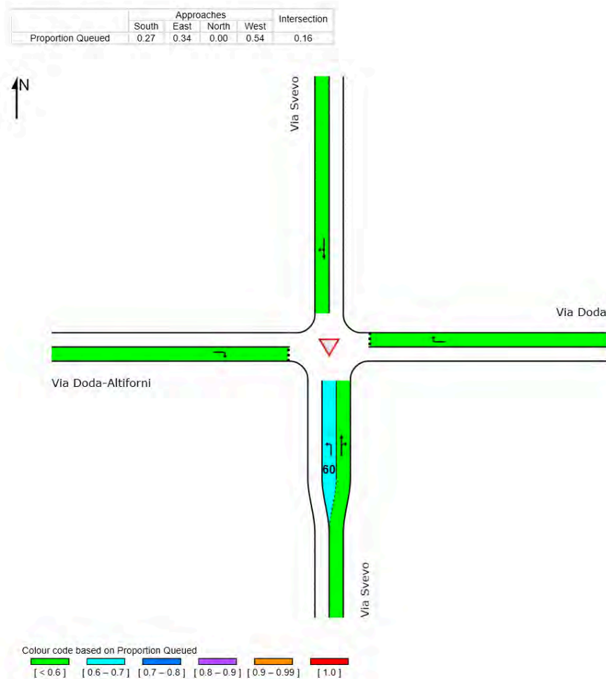
Figura 20 – Proporzioe di traffico in coda – Scenario di cantiere B
