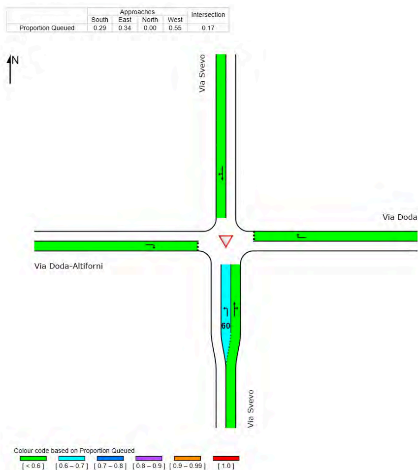
Figura 18 – Proporzioe di traffico in coda – Scenario di cantiere A
