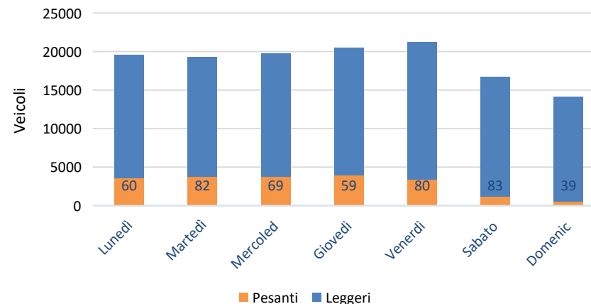
Veicoli giornalieri medi
