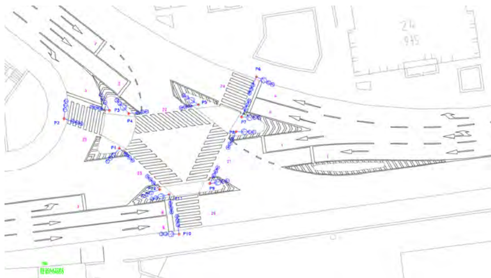
Figura 7 - Layout dell'intersezione K47 con denominazione dei relativi segnali semaforici
