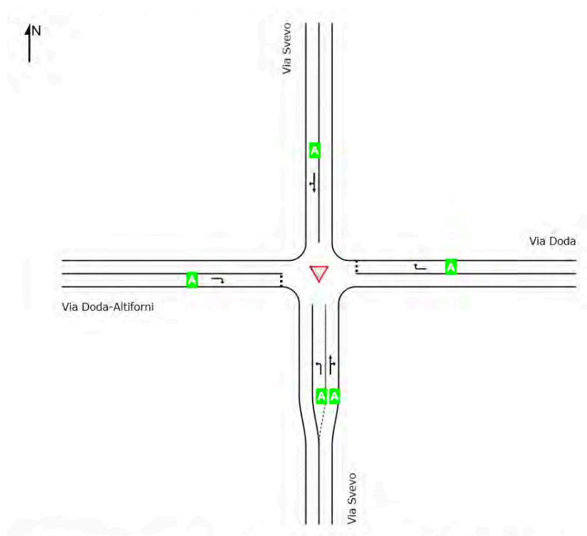
Figura 19 – Livello di Servizio per corsia – Scenario di cantiere B
