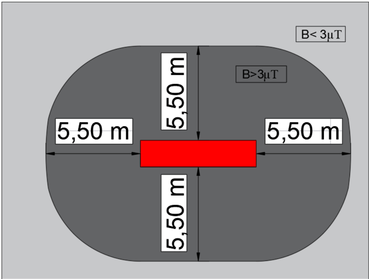
Figura 18: indicazione della DPA delle cabine elettriche di conversione e trasformazione dell'energia elettrica prodotta valutata applicando la procedura prevista dal DM 29 maggio 2008
