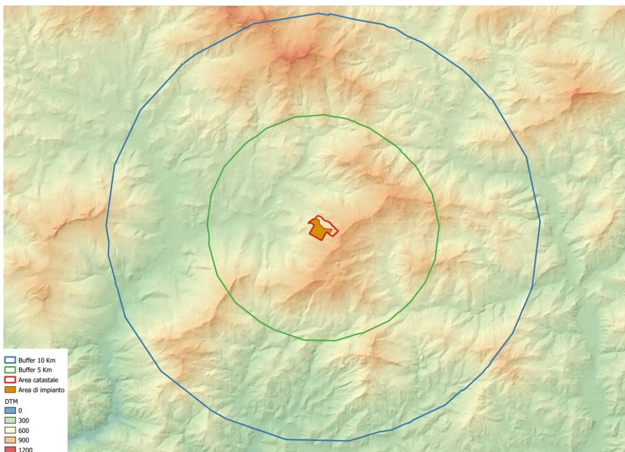
Figura 15 - elaborazione carta della visibilità su DTM
