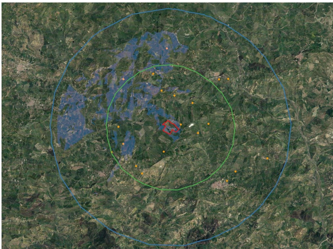
Figura 16 - Mappa intervisibilità su ortofoto
