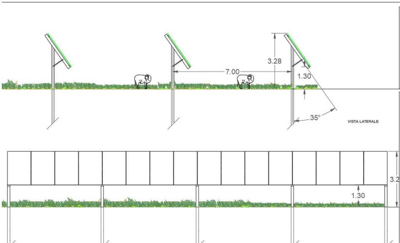
Figura 4 - vista laterale e frontale delle strutture fisse
