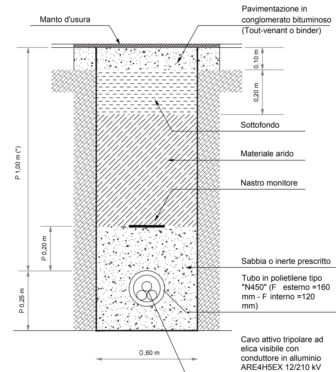
LINEA IN CAVO SOTTERRANEO IN TUBAZIONE POSA DI N.1 CAVI AT IN STRADA COMUNALE ASFALTATA
