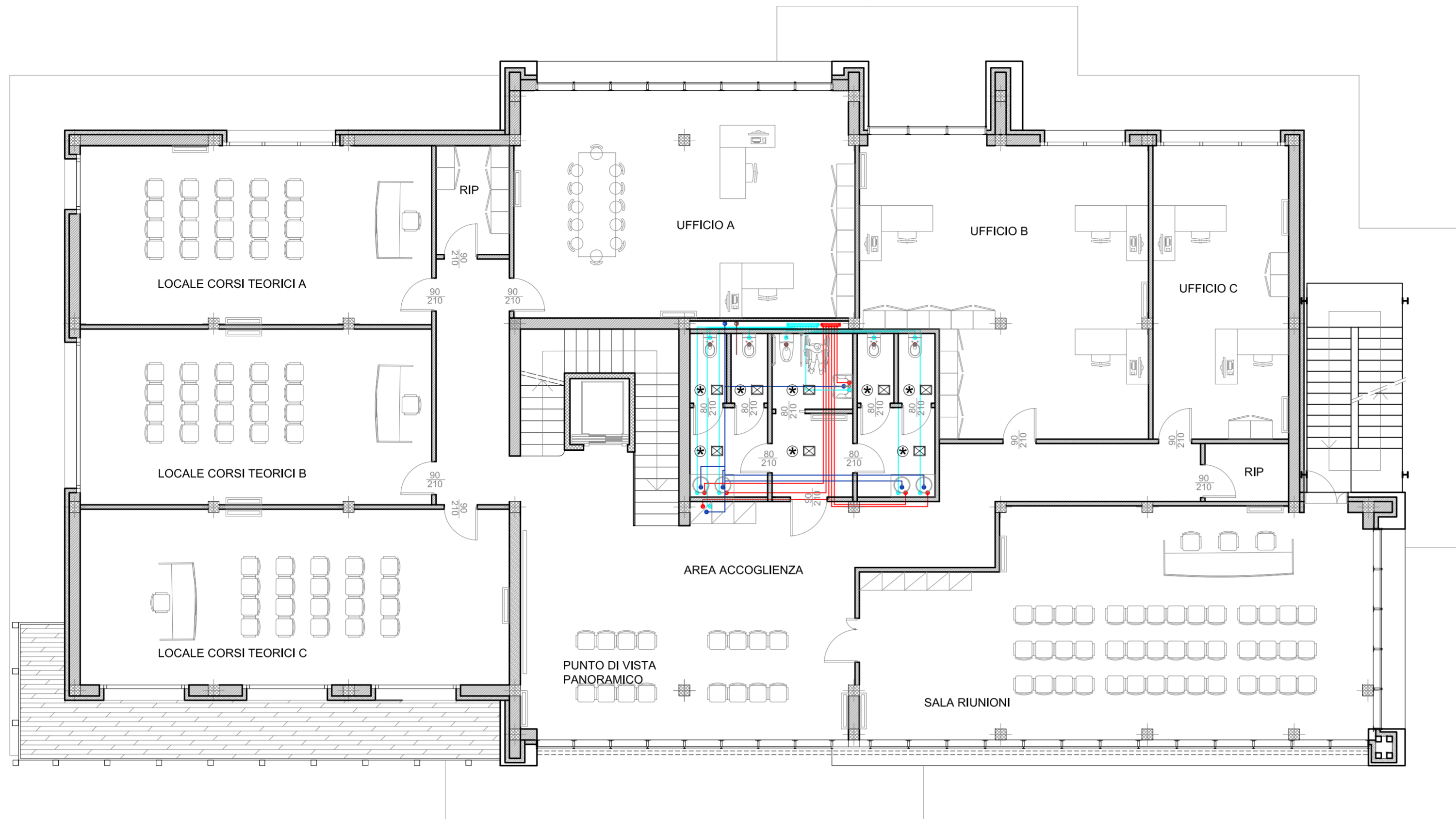
PIANTA PIANO PRIMO schema impianto idrico sanitario - scala 1:100 quote in cm
