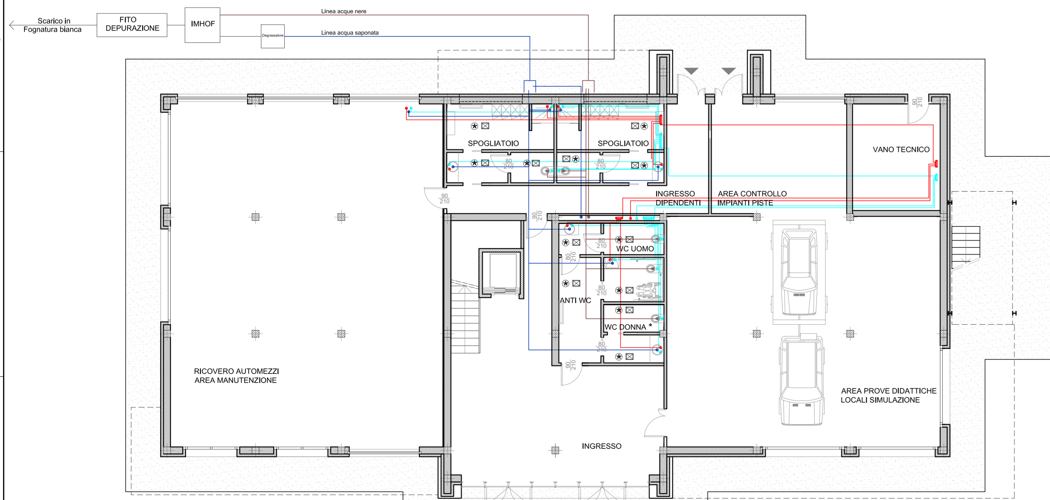
PIANTA PIANO TERRENO schema impianto idrico sanitario - scala 1:100 quote in cm
