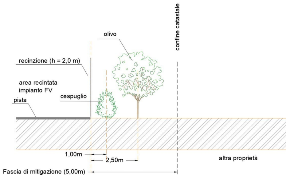
Figura 2.12. – Stralcio di sezione dell'area perimetrale dell'impianto.
