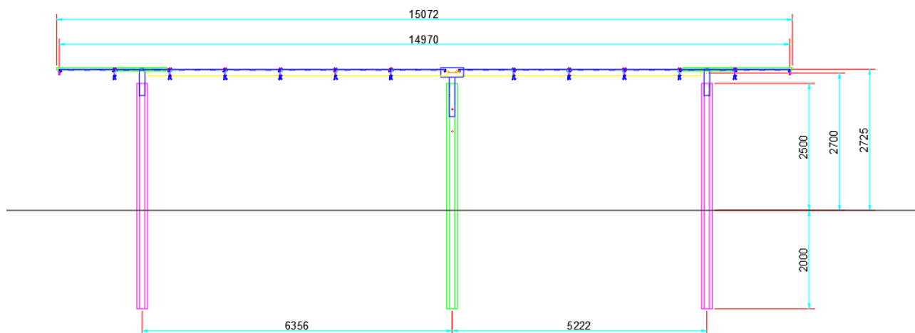
Figura 2.4 – Sezione longitudinale.
