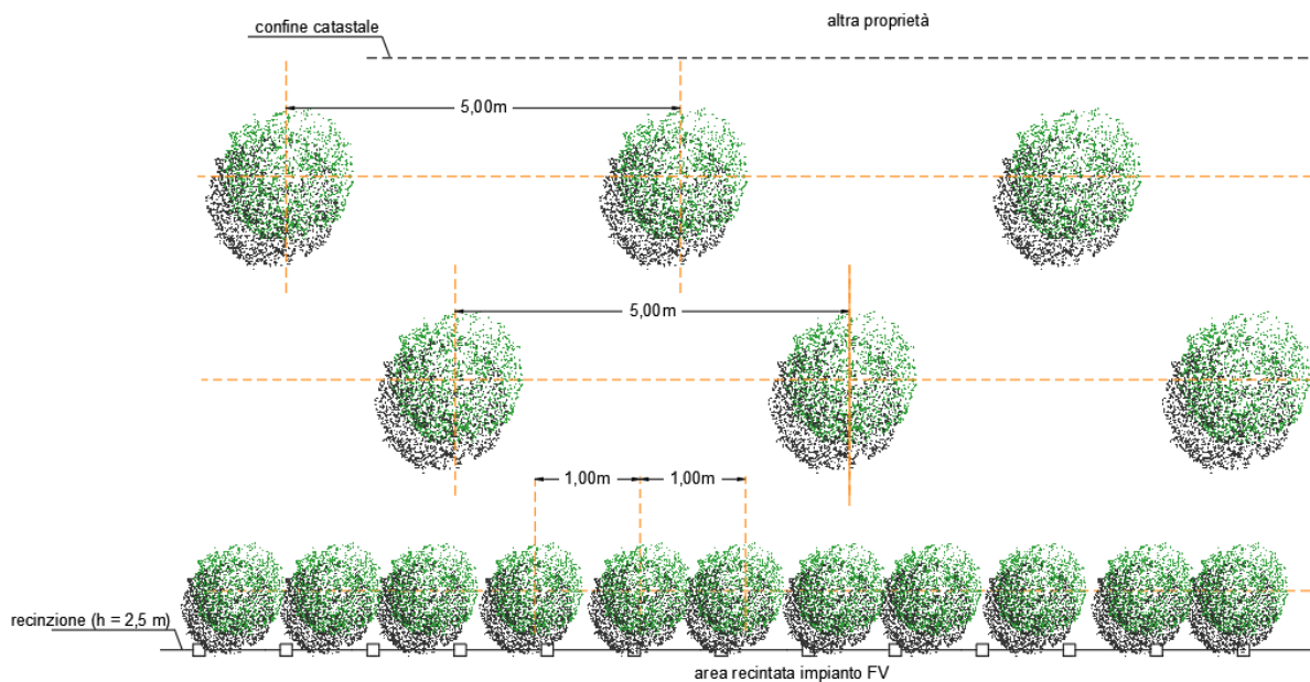
2.14 – Siepe polispecifica (planimetria di progetto).
