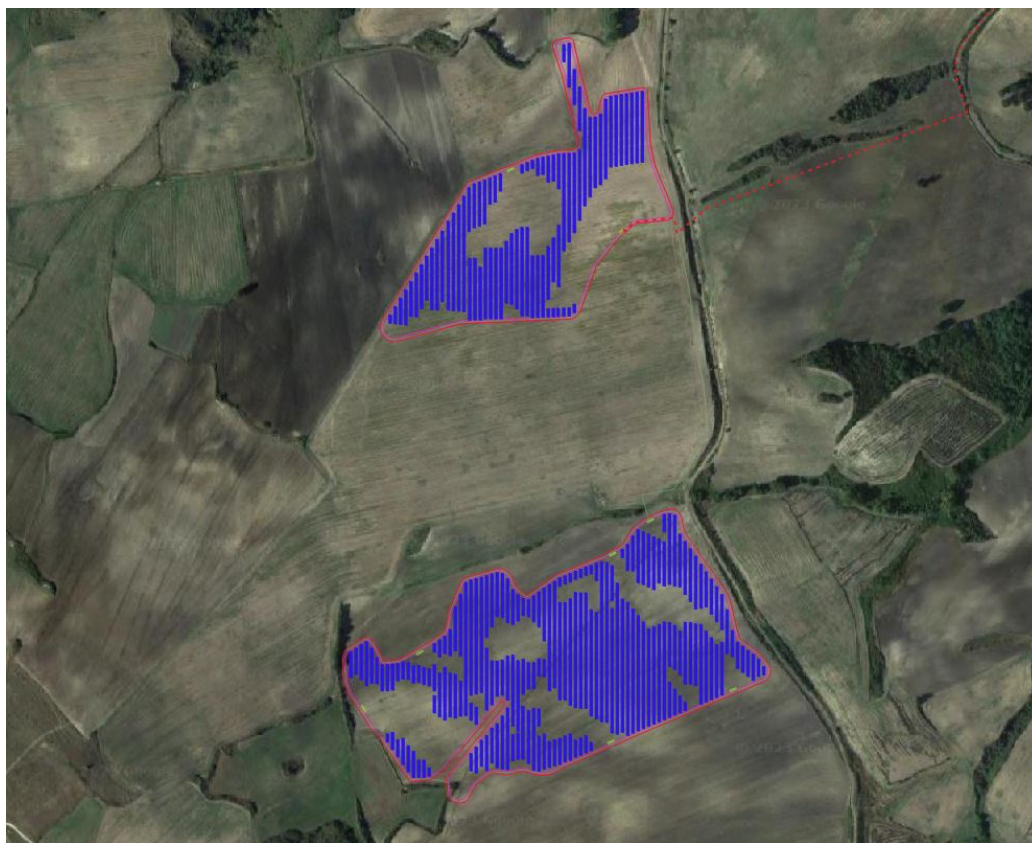
Figura 4.2. – Layout del sistema agrivoltaico con tracker.
