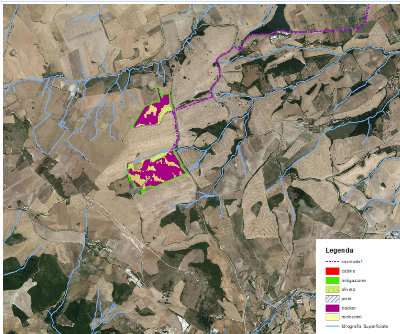
Figura 1.11 Idrografia dell'area
