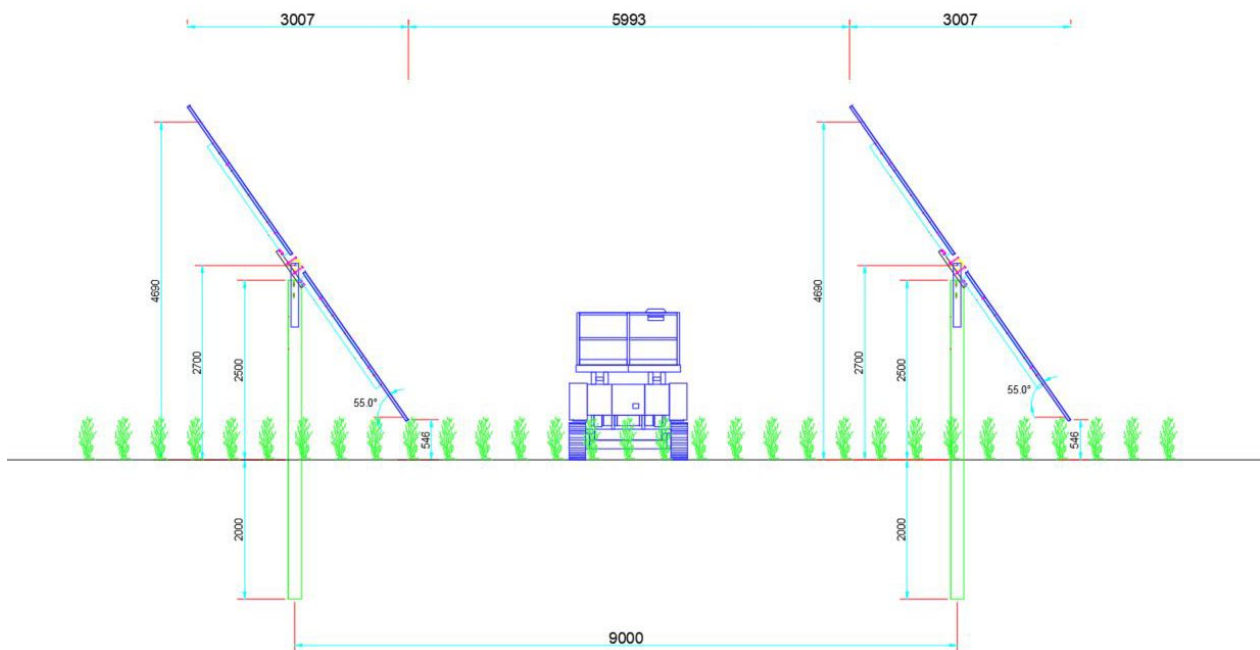
Figure 12.8. – Sezione tipo Aree coltivate.
