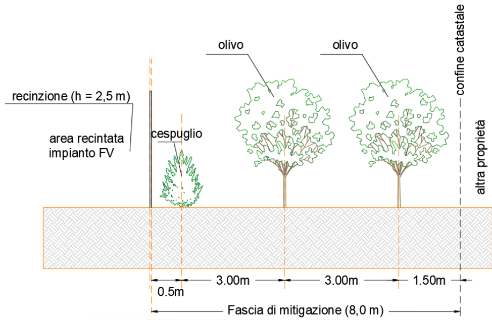
Figura 12.6. – Stralcio di sezione dell'area perimetrale dell'impianto.
