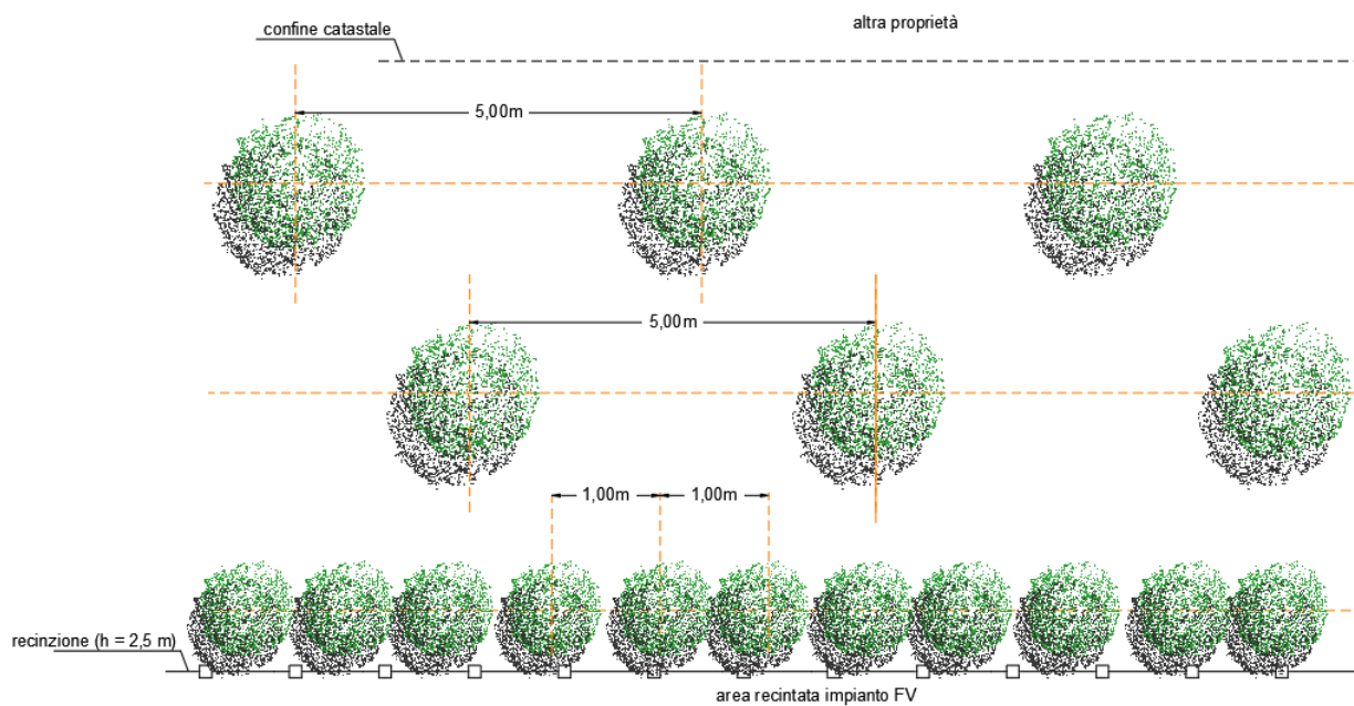
Figura 12.5. – Siepe polispecifica (planimetria di progetto).
