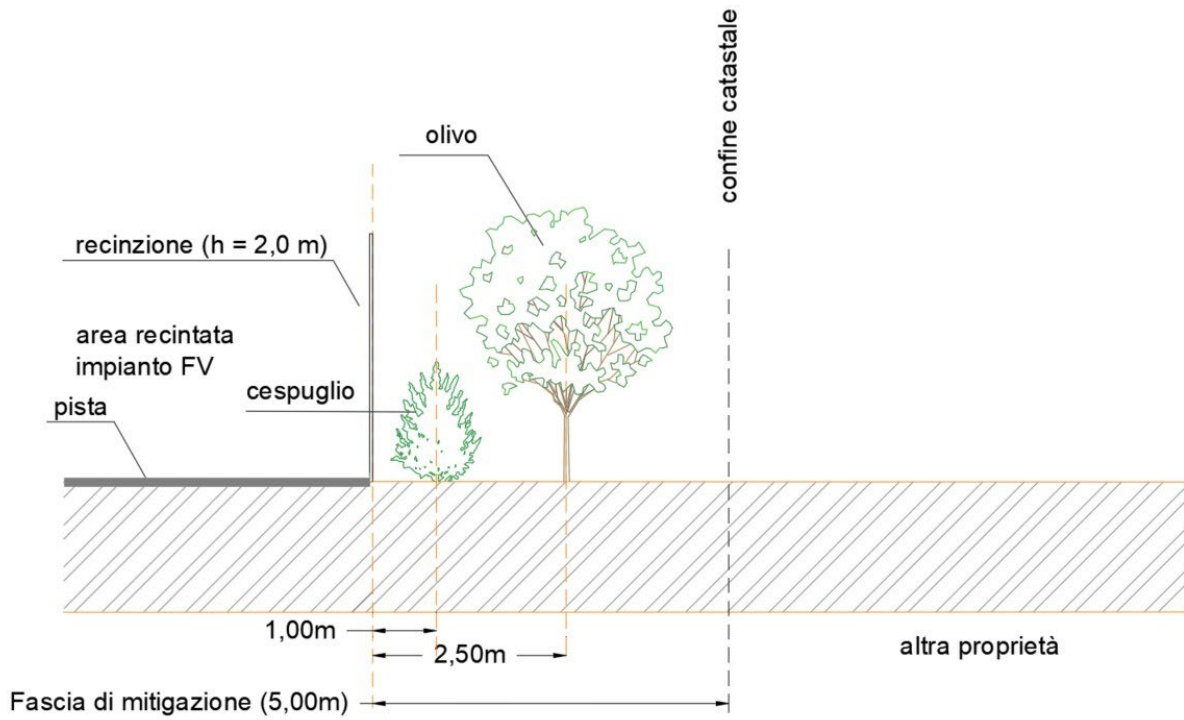
Figura 12.3. – Stralcio di sezione dell'area perimetrale dell'impianto.
