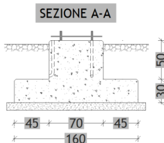
Fig. Pianta e sezione fondazione per scaricatore AT
