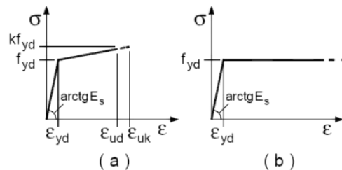
Diagrammi di calcolo tensione/deformazione dell'acciaio.
