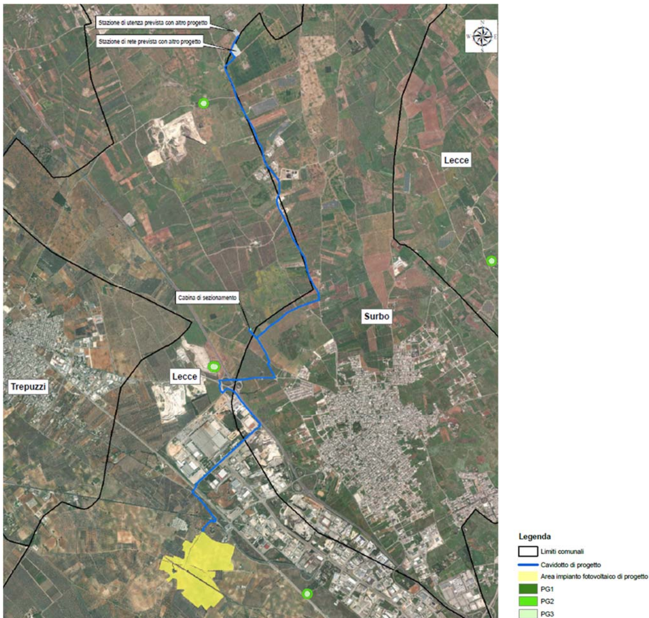
Figura 6 - Inquadramento area impianto su aree a pericolosità geomorfologica
