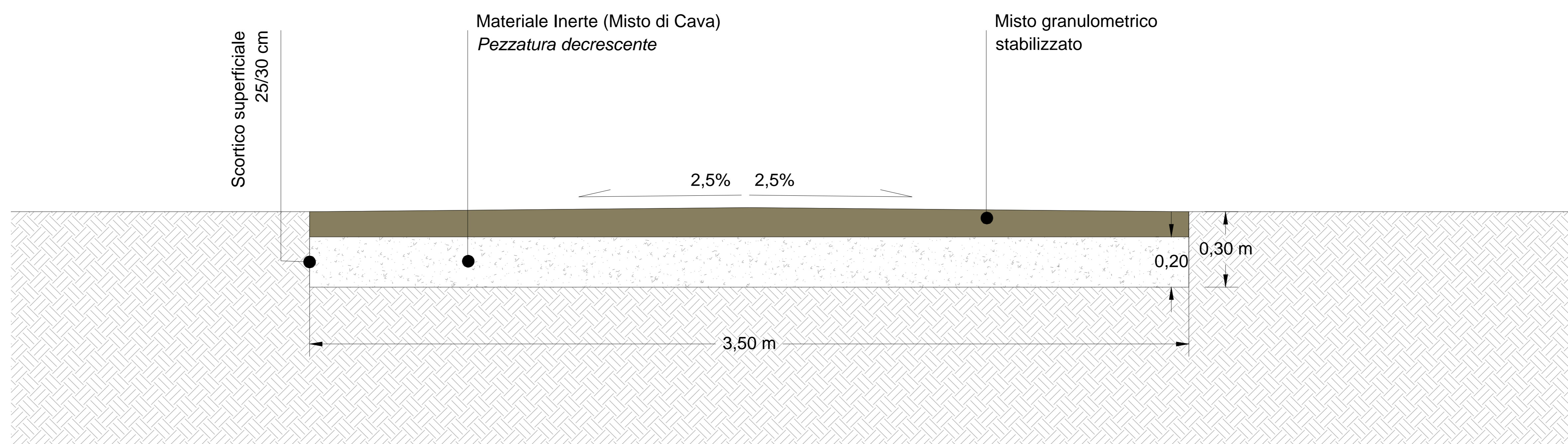
Particolare viabilità' interna - scala 1:10
