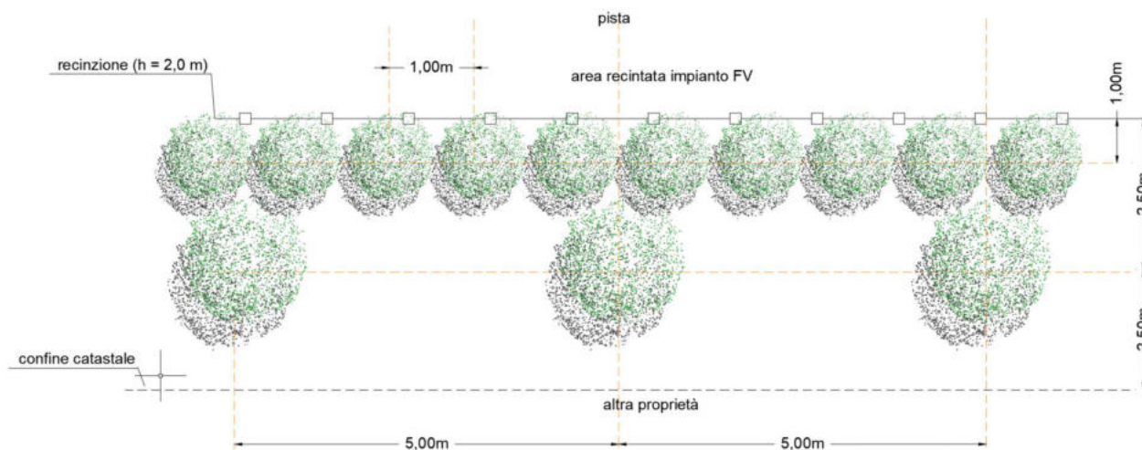
Figure 14.3. – Sezione polispecifica (planimetria di progetto).
