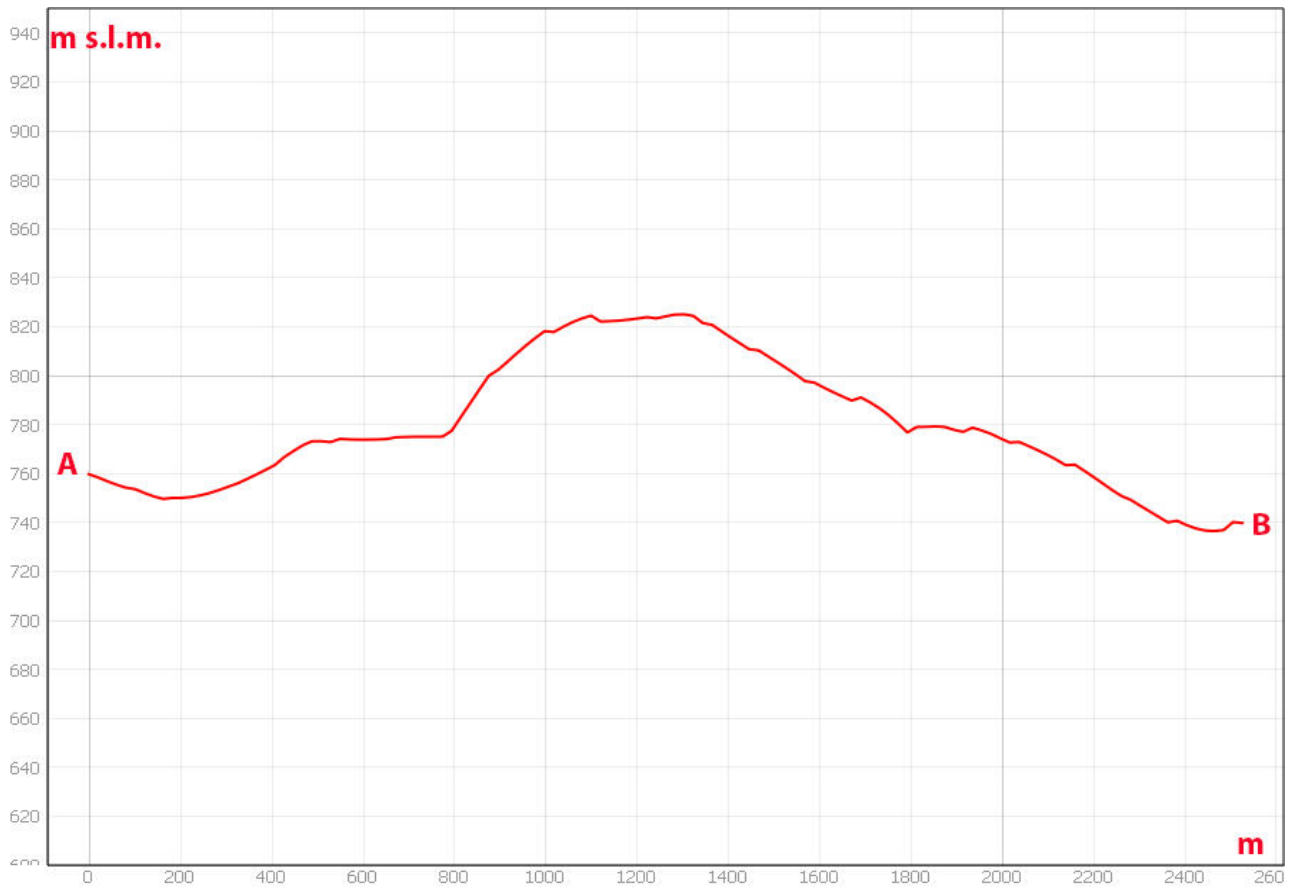
Sezione morfologica del terreno- Punto di presa n°16
