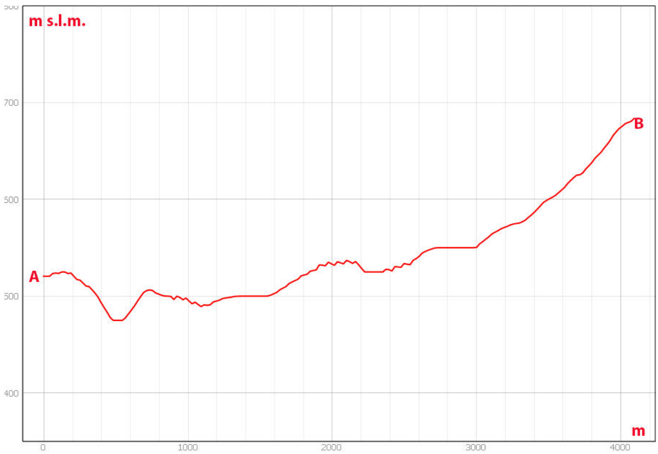
Sezione morfologica del terreno- Punto di presa n°9
