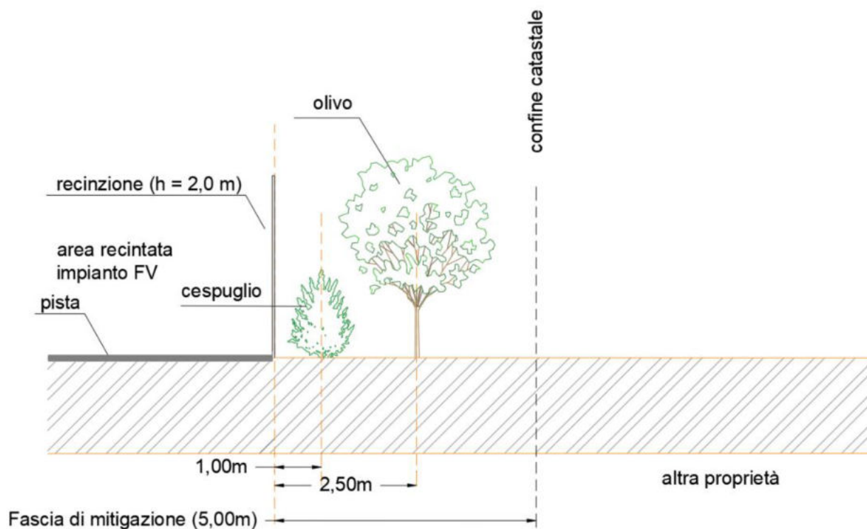
Figure 14.4. – Stralci di sezione dell'area perimetrale dell'impianto.
