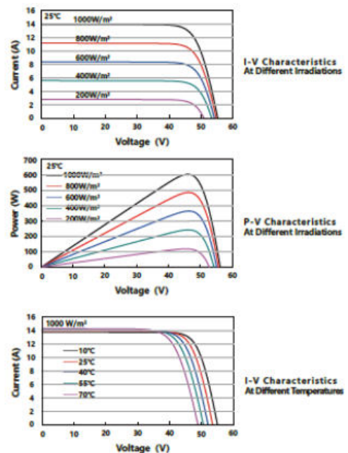
Figura 6.5. – Scheda tecnica del modulo fotovoltaico della JOLYWOOD, modello JW-HD156N BIFACIAL.
