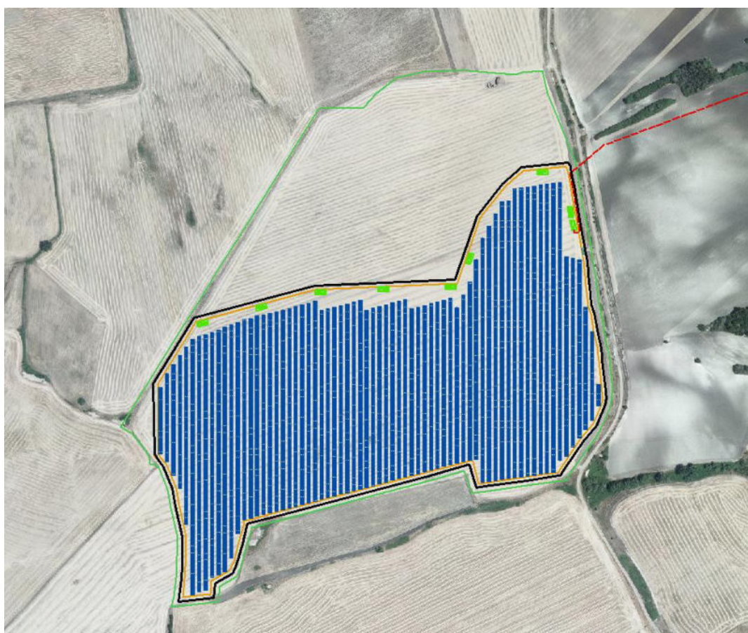
Figura 7.1. – Layout del sistema agrivoltaico con tracker.
