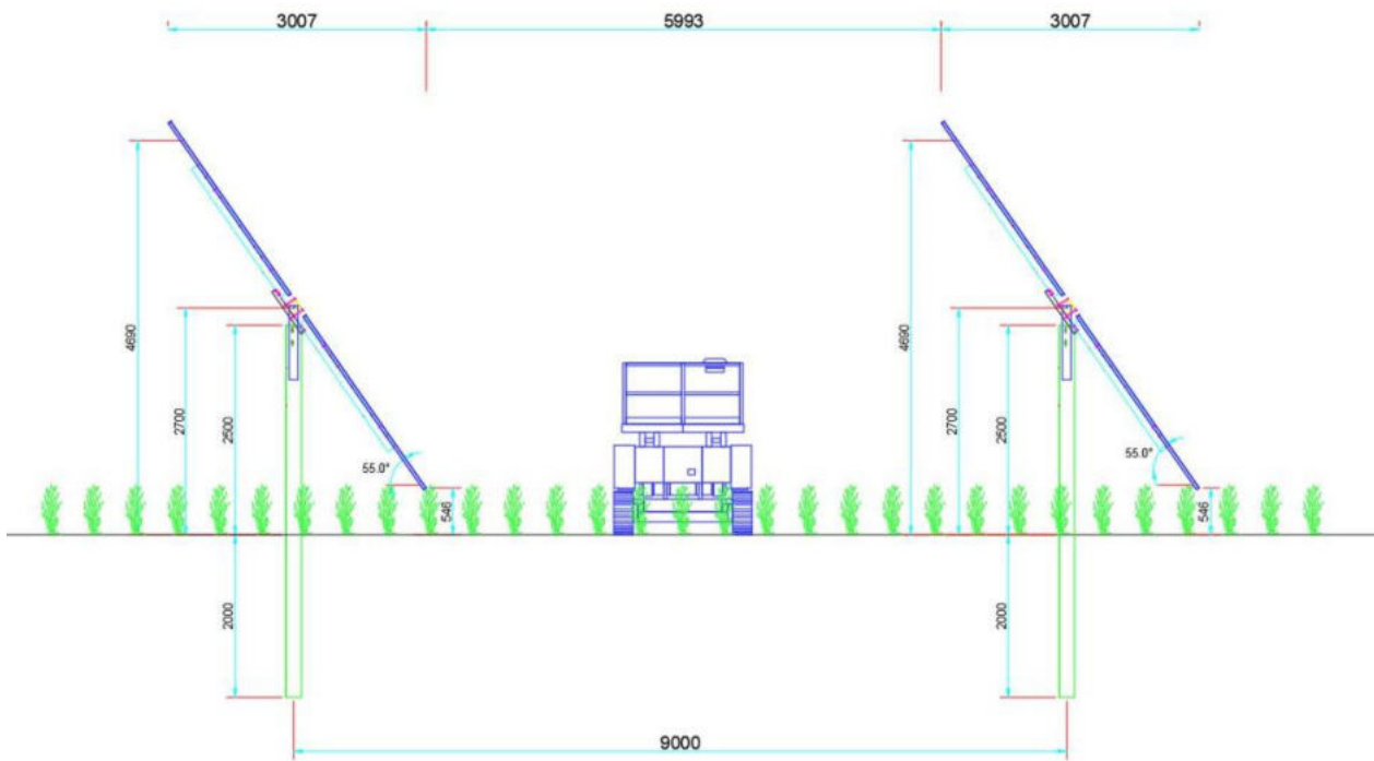
Figura 6.7. – Struttura di supporto con distanza tra i tracker e coltivazione sottostante.
