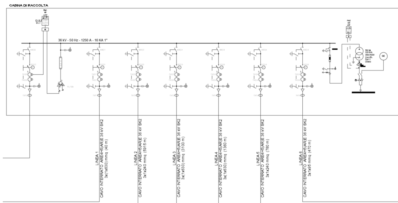
Schema della cabina di consegna
