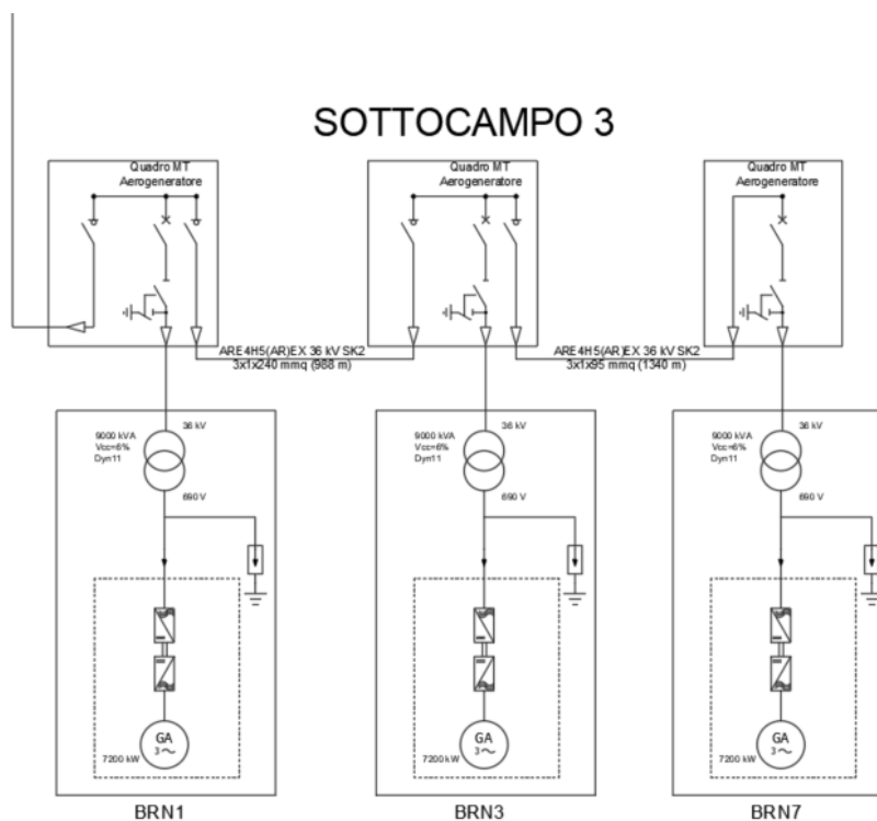
Schema a blocchi del parco eolico GRUPPO 3
