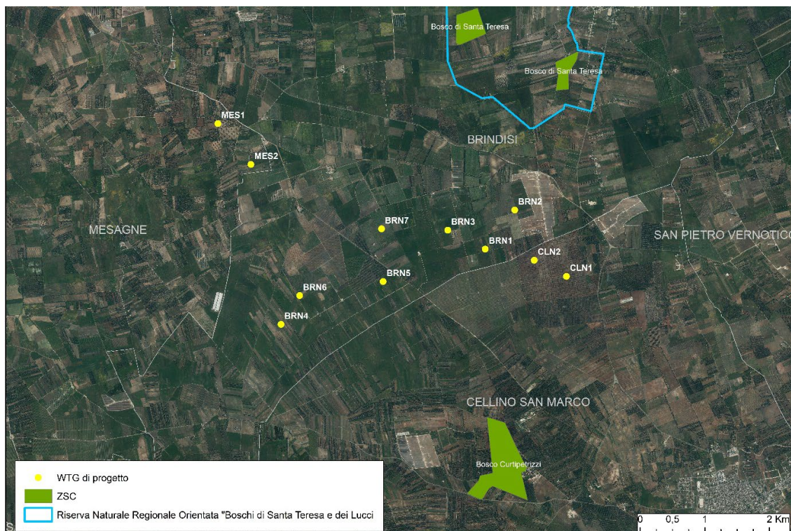
Aerogeneratori di progetto, aree naturali protette e Natura 2000.
