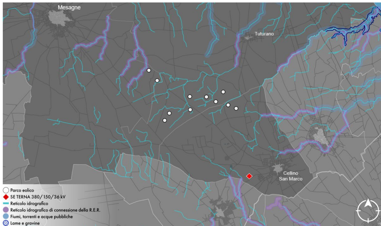
Struttura idro-geomorfologica
