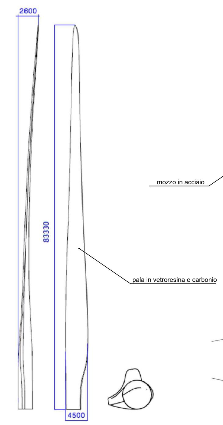
scala 1:500
