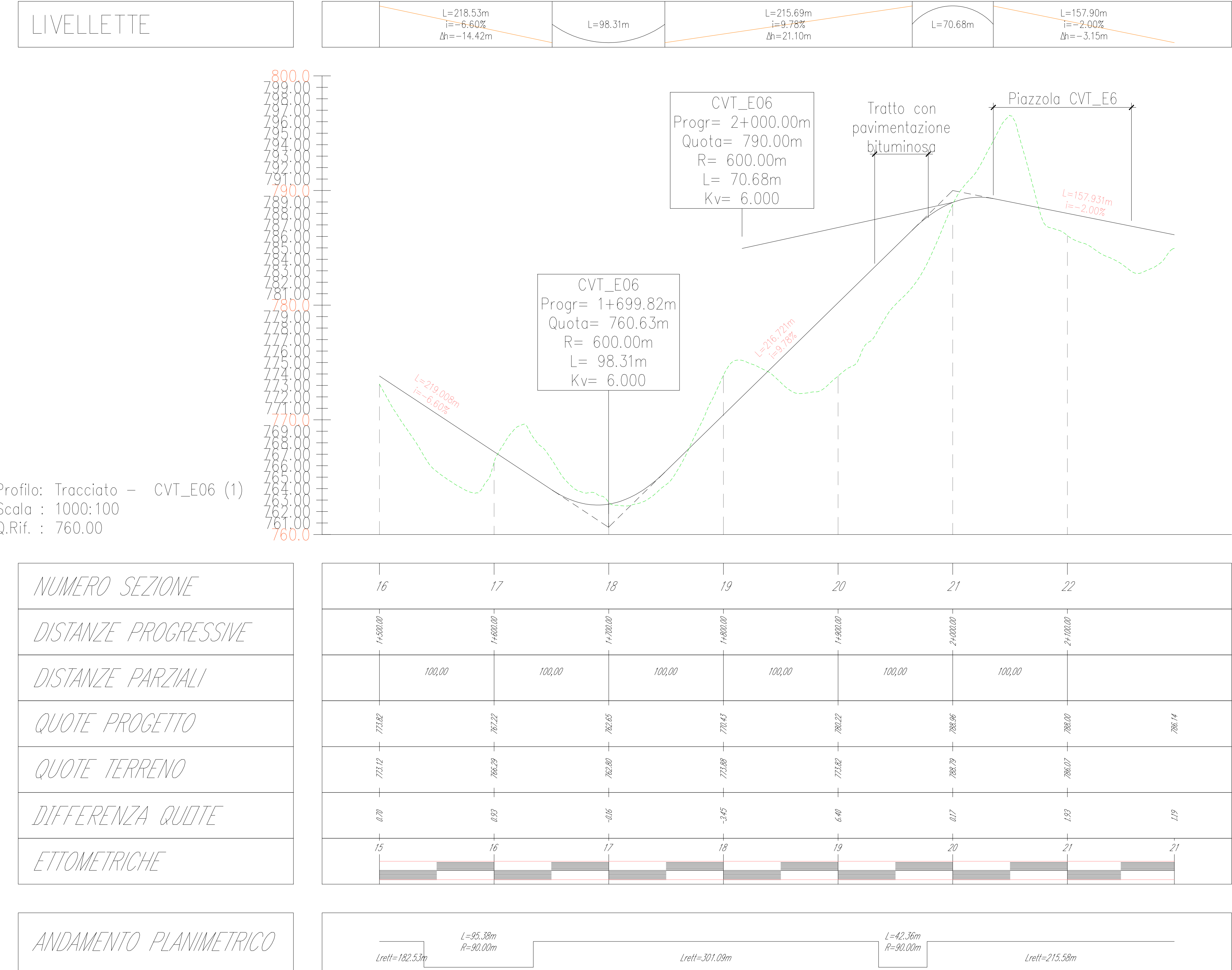
PROFILO - Scala 1:2.000
