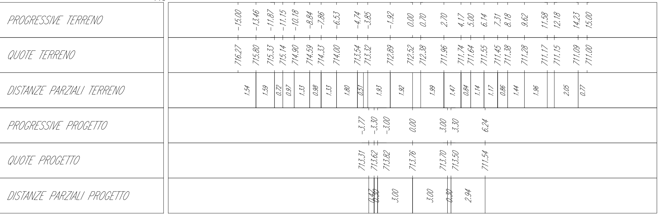
Tracciato - CVT_E8 Sez. 18 Progr.: 1+700.00 Scala : 1:2000 Q.Rif. : 710.00
