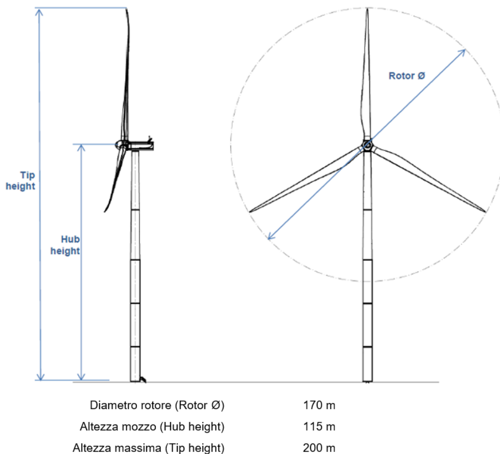
Figura 3-3: Vista e caratteristiche di un aerogeneratore da 4,52 MW
