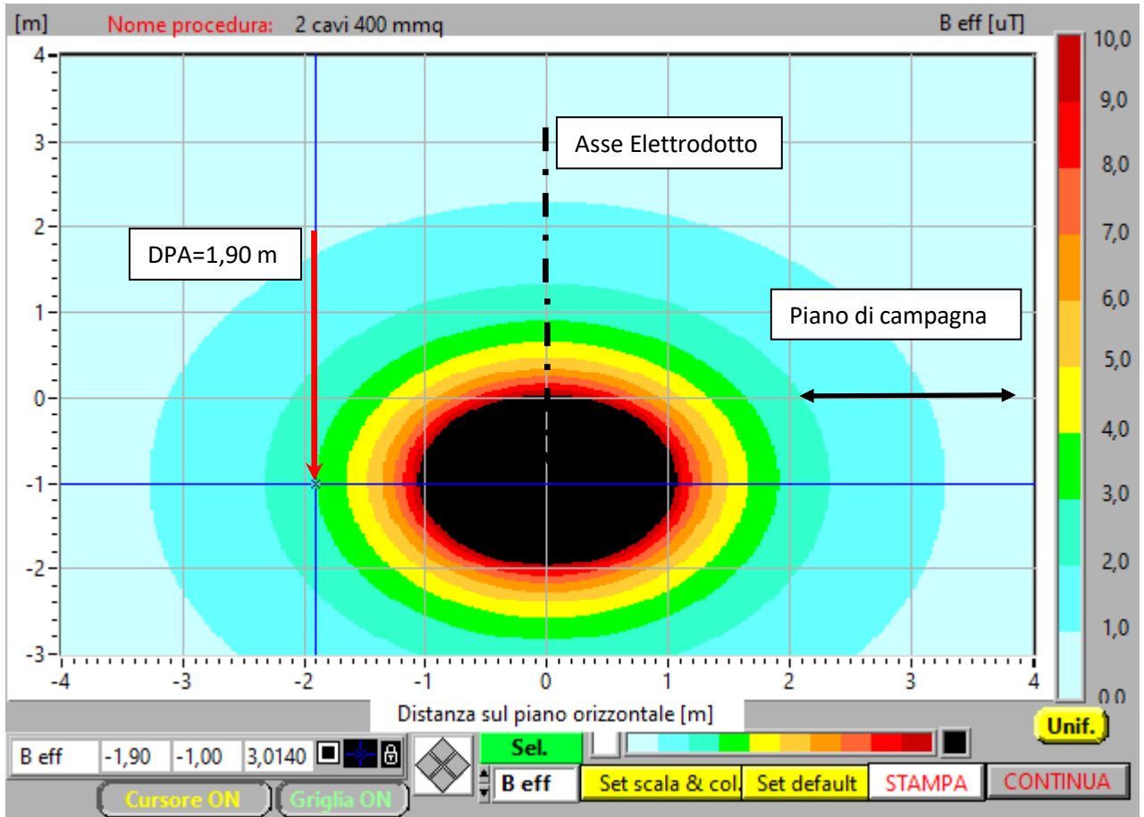
Figura 8. Mappa verticale induzione magnetica (B) sezione tipo con indicazione della DPA - V=30 kV I = 231 A
