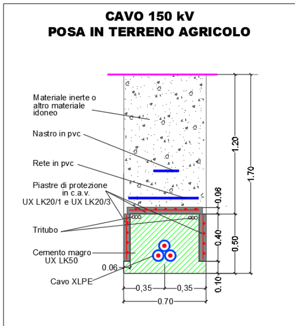
Figura 20. Posa cavo 150 kV "SE 30/150 kV-SE 380/150 kV TERNA SATELLITE in AVETRANA(TA)"
