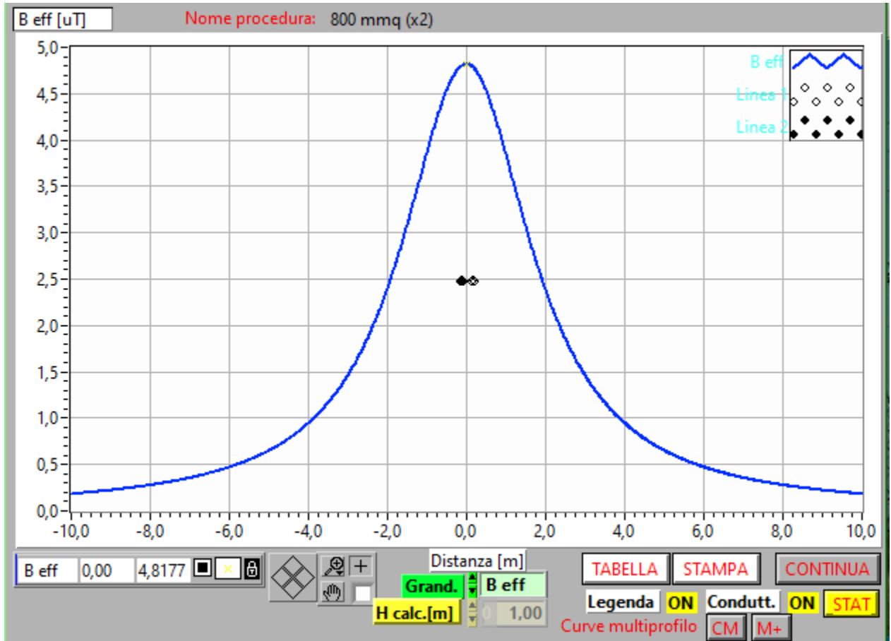
Figura 11. Profilo laterale induzione magnetica (B) sezione tipo con indicazione della DPA - V=30 kV I = 347 A
