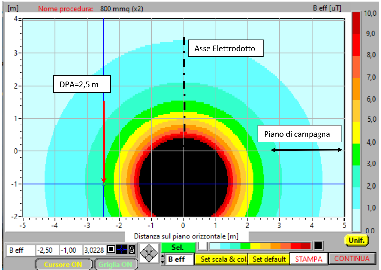
Figura 12. Mappa verticale induzione magnetica (B) sezione tipo con indicazione della DPA - V=30 \text{ kV} I = 347 \text{ A}
