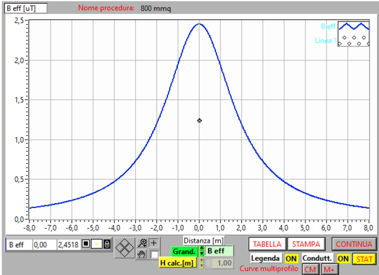
Figura 5. Profilo laterale induzione magnetica (B) sezione tipo con indicazione della DPA - V=30 kV I = 347 A
