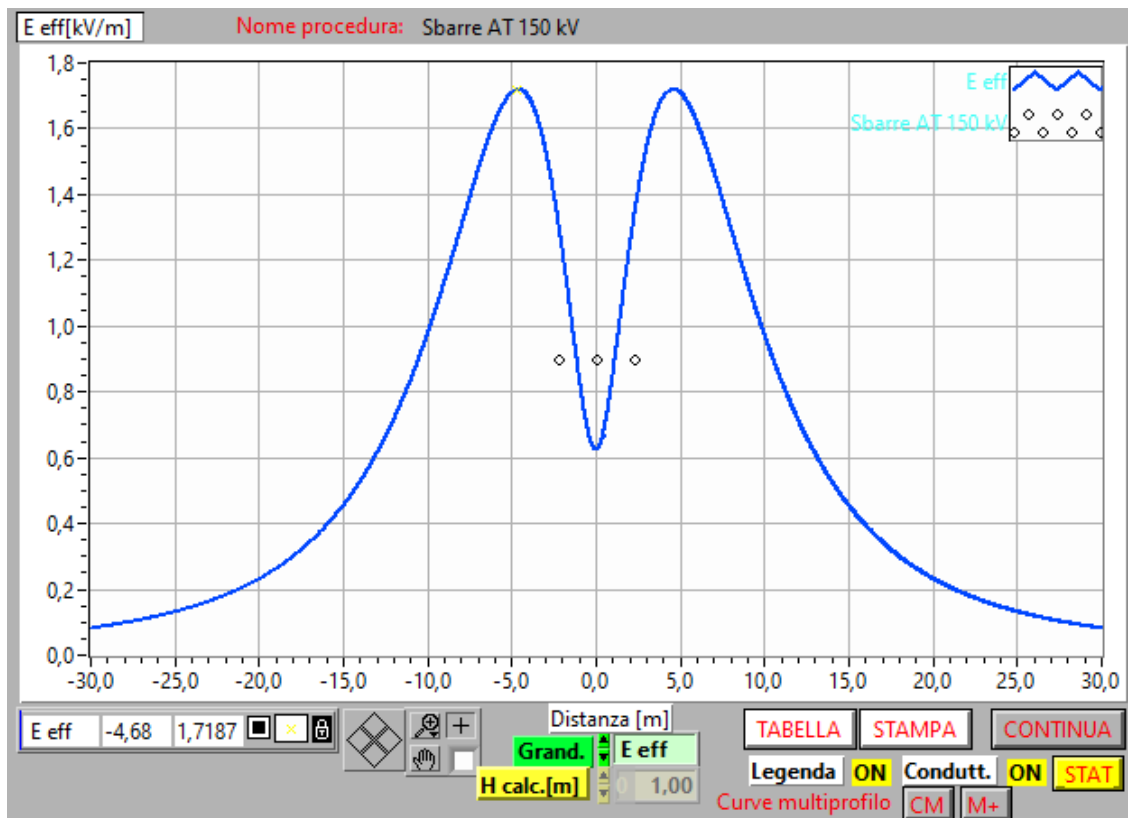
Figura 24. Profilo laterale campo elettrico (E) sbarre 150 kV
