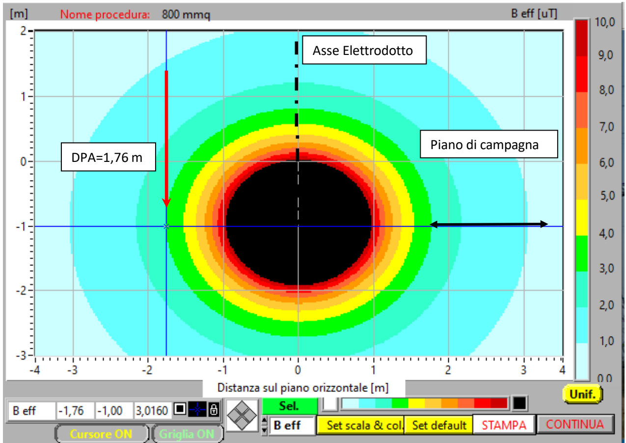
Figura 6. Mappa verticale induzione magnetica (B) sezione tipo con indicazione della DPA - V=30 \text{ kV} I = 347 \text{ A}
