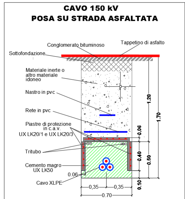
Figura 20. Posa cavo 150 kV "SE 30/150 kV-SE 380/150 kV TERNA SATELLITE in AVETRANA(TA)"
