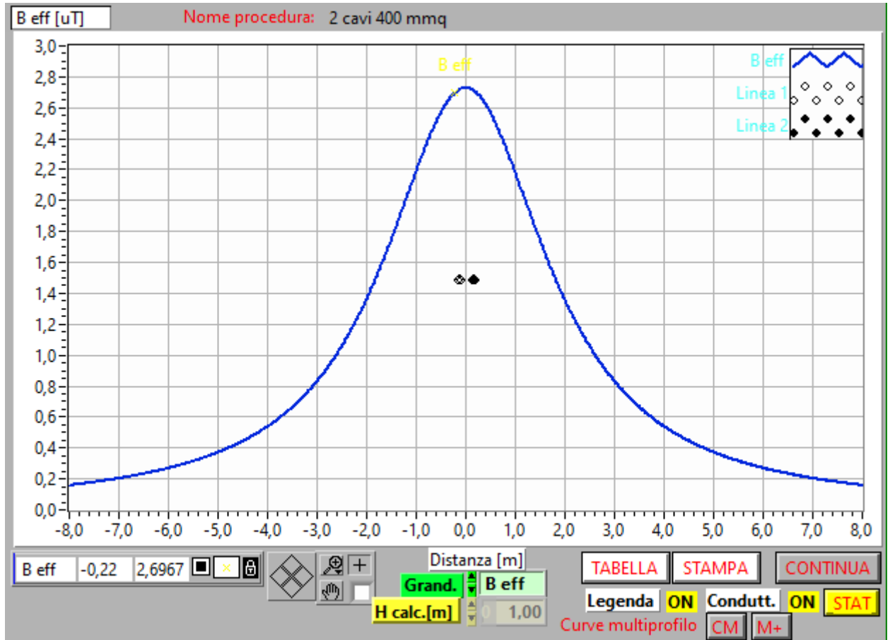
Figura 7. Profilo laterale induzione magnetica (B) sezione tipo con indicazione della DPA - V=30 kV I = 231 A
