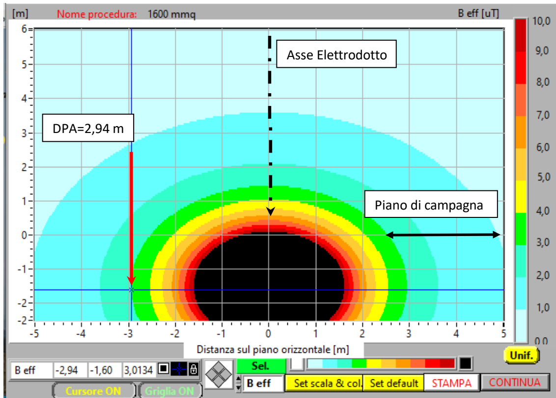
Figura 22. Mappa verticale induzione magnetica (B) sezione tipo con indicazione della DPA - V=150 \text{ kV} I=1000 \text{ A}
