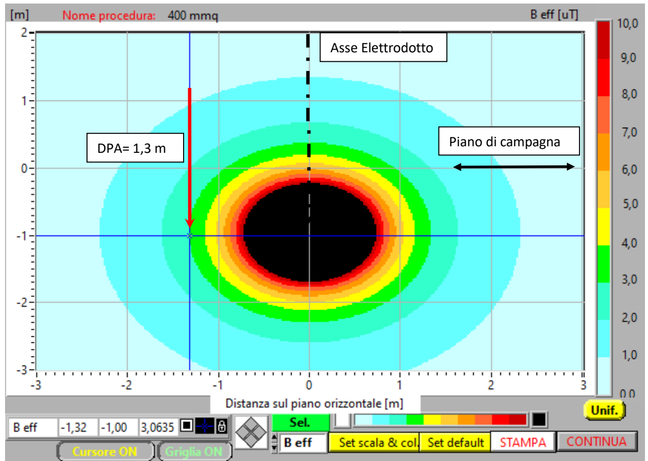
Figura 4. Mappa verticale induzione magnetica (B) sezione tipo con indicazione della DPA - V=30 \text{ kV} I = 231 \text{ A} ; P=12\text{MW}
