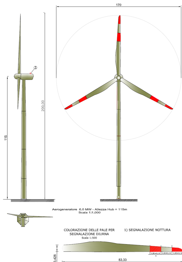
Fig.5 Vista e caratteristiche dell'aerogeneratore di riferimento – SG170-6,0
