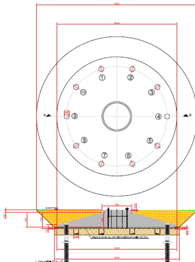
Figura 11- Pianta-sezioni e armature del plinto di fondazione
