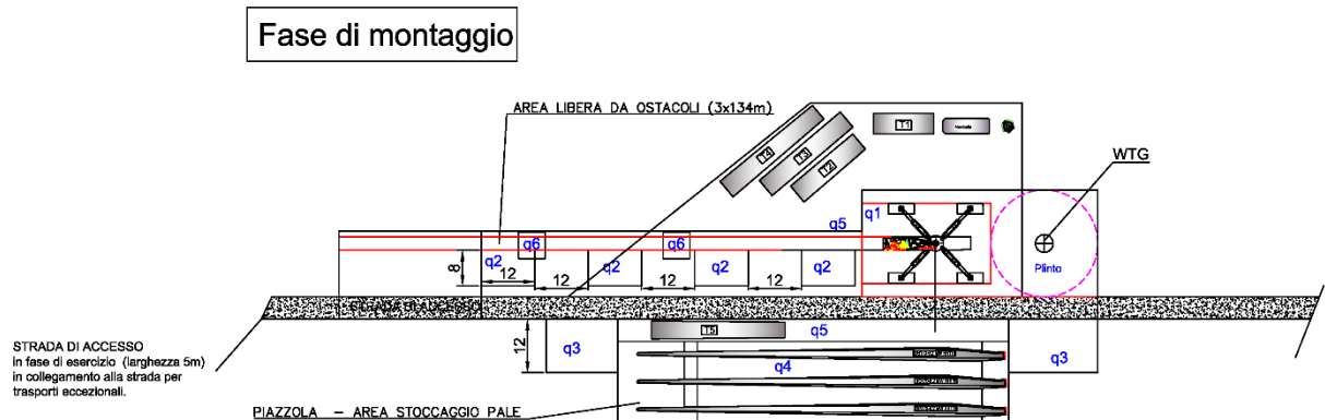
Figura 9: Piazzola montaggio aerogeneratore con component
