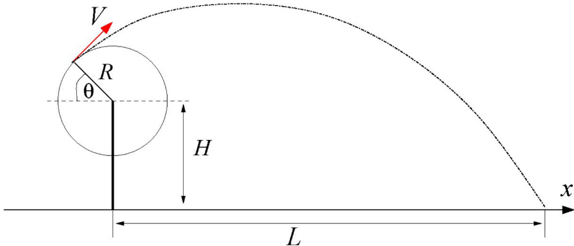
Fig.7 – Schema gittata
