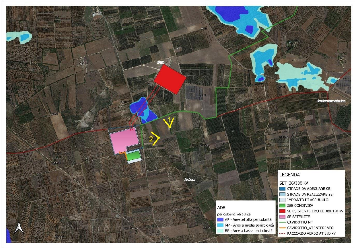
Figura 12: Area SSE NEXT2 con futura SE SATELLITE nel Comune di Avetrana(Ta)
