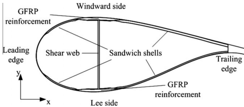
Tipica sezione trasversale di una pala eolica 1
