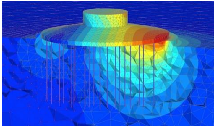
Figura 10- Schema tridimensionale di fondazione – Plinto su pali
