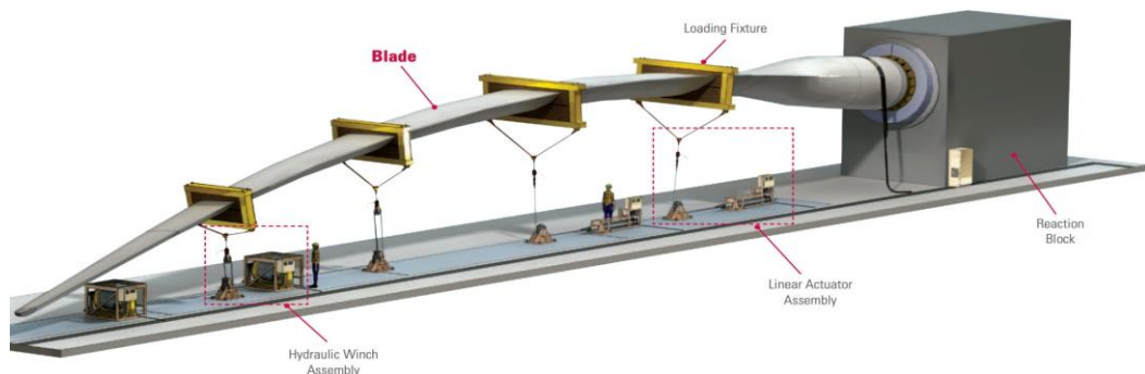
Prova statica su una pala di turbina eolica a scala reale 2
