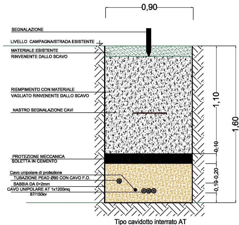
Figura 15. Posa cavo 150 kV "SE 30/150 kV-SE 380/150 kV TERNA Cellino San Marco"
