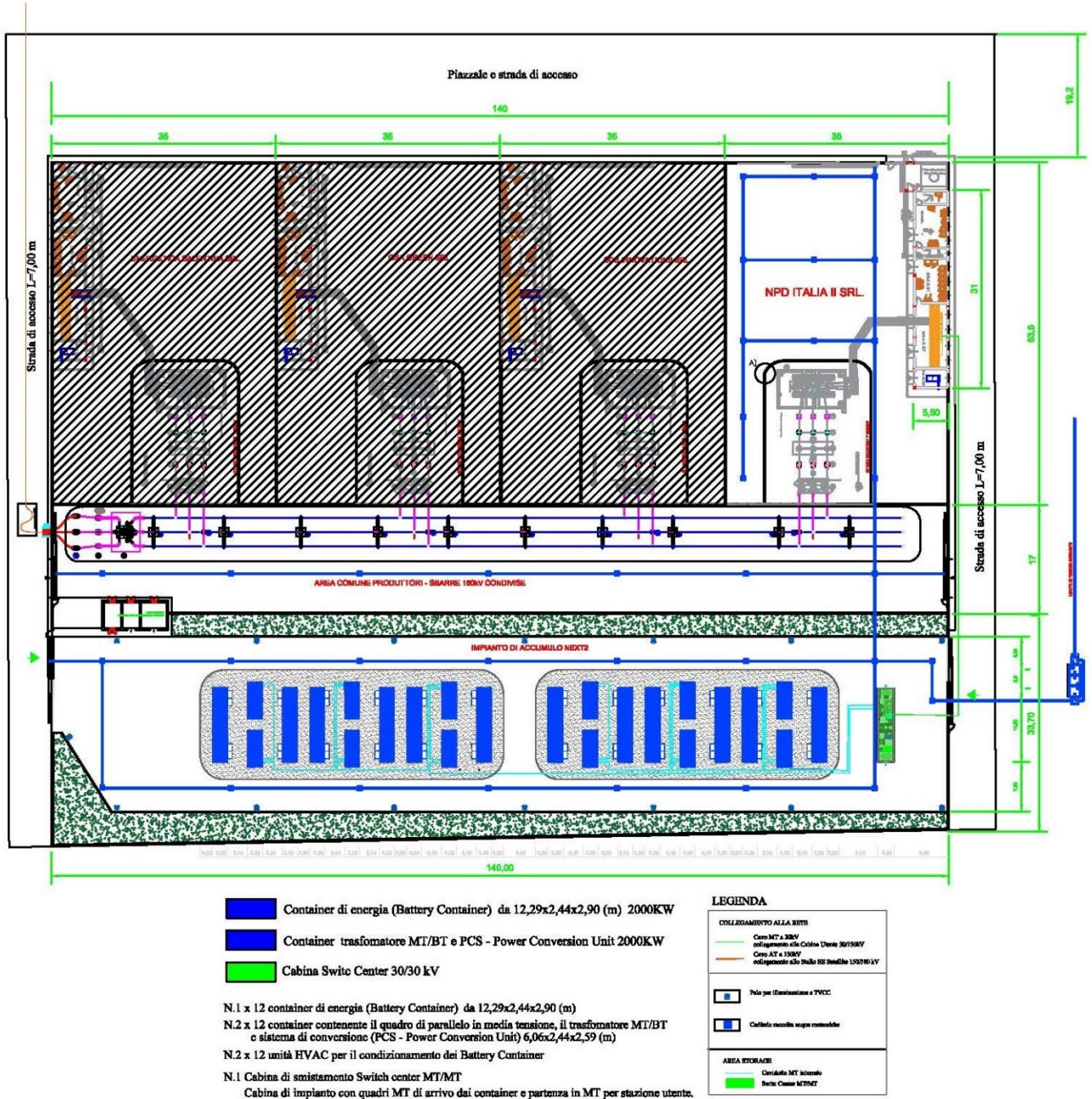
Figura 14: Planimetria SSE con area a sbarre (in rosso la cabina NEXT2)
