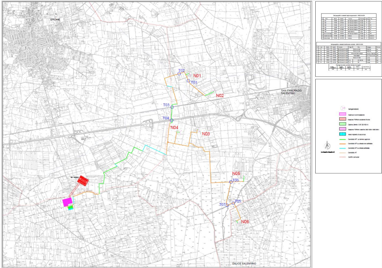
Figura – Inquadramento parco eolico con indicazione delle tipologie di attraversamenti previsti(CFR-_CTR_1_05a) Nell’elaborato grafico 1_05b-1 sono riportati i report fotografici in sito delle aree oggetto di TOC.
