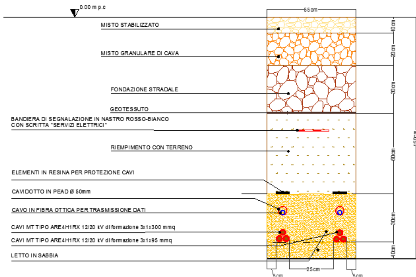
Fig. 5. Rappresentazione della Linea di Esplorazione del campo magnetico rispetto ad un elettrodotto interrato tipo.
