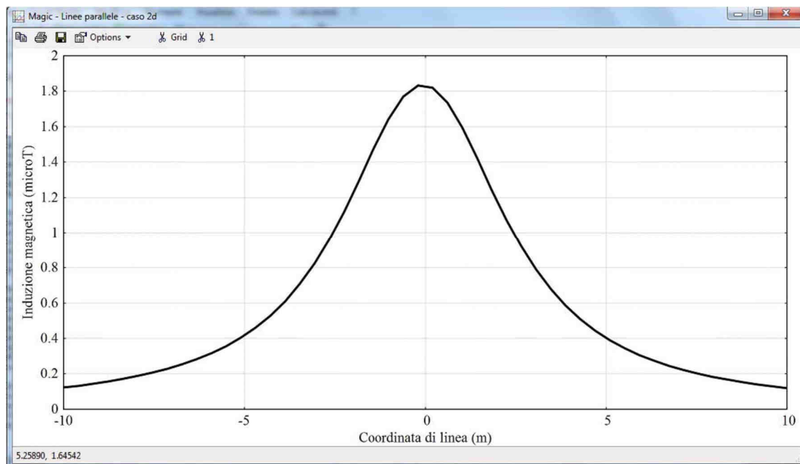
Fig. 11. Rappresentazione bidimensionale dei risultati il cui riferimento di calcolo dell'induzione magnetica è a quota pari alla linea di esplorazione (Fig. 4)
