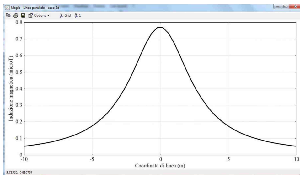
Fig. 7. Rappresentazione bidimensionale dei risultati il cui riferimento di calcolo dell'induzione magnetica è a quota pari alla linea di esplorazione (Fig. 4)
