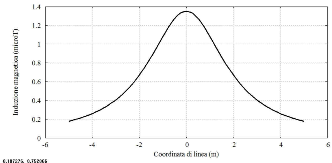
Fig. 9. Rappresentazione bidimensionale dei risultati il cui riferimento di calcolo dell'induzione magnetica è a quota pari alla linea di esplorazione (Fig. 4)
