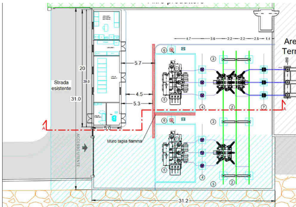
Fig. 1 Planimetria elettromeccanica dello stallo di progetto
