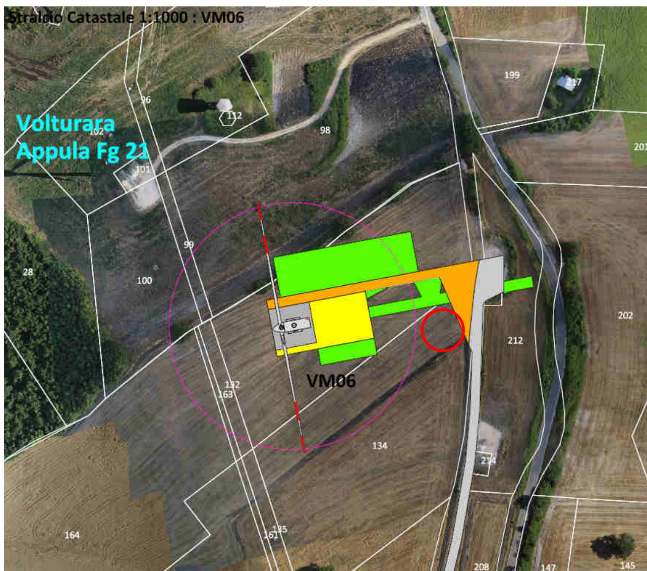
Fig. 2. Area della stazione metereologica (cerchio rosso)
