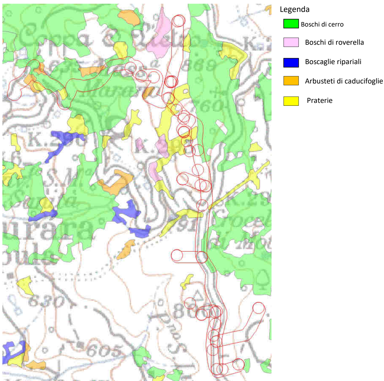
Fig. 3- Carta della vegetazione di origine spontanea
