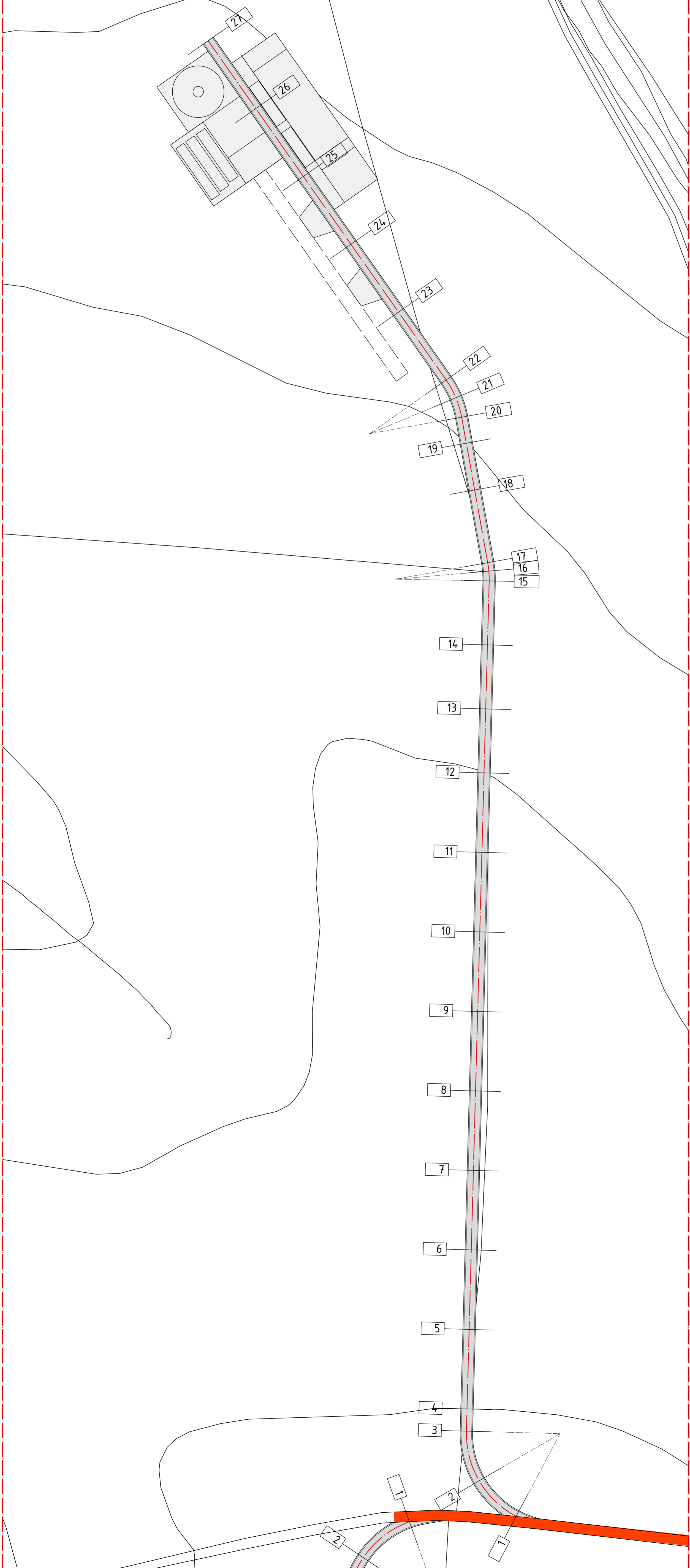
Planimetria WTG-B Scala 1:1.000
