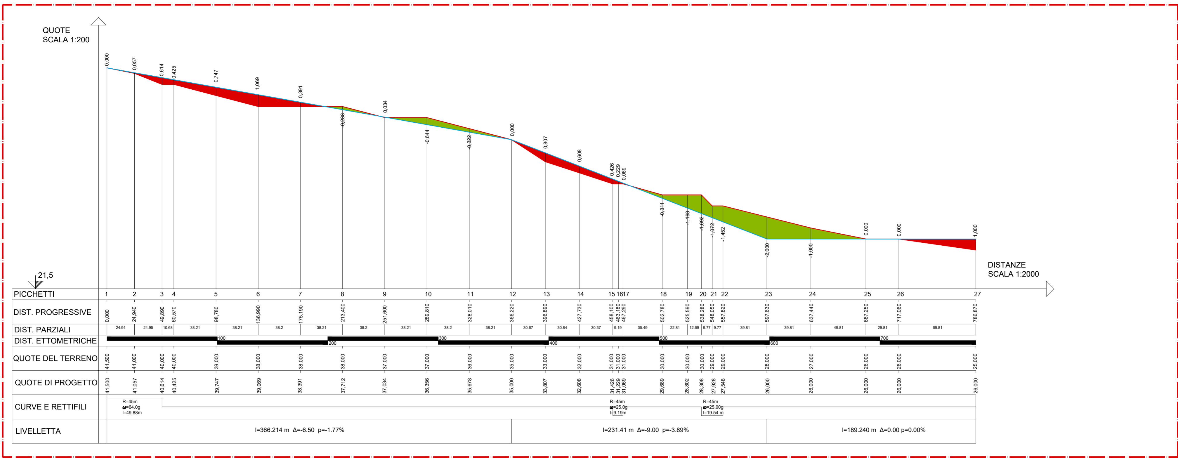
Profilo altimetrico WTG-B Scala 1:2.000
