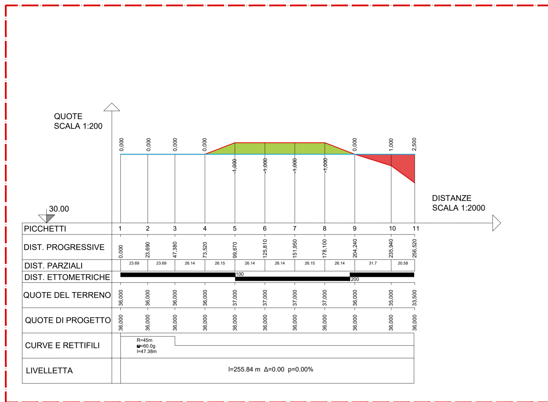
Profilo altimetrico WTG-C Scala 1:2.000
