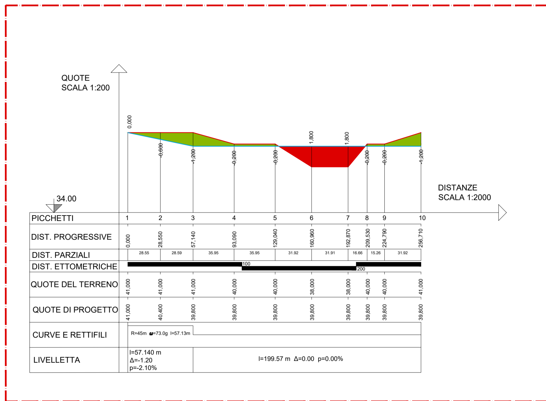
Profilo altimetrico WTG-D Scala 1:2.000
