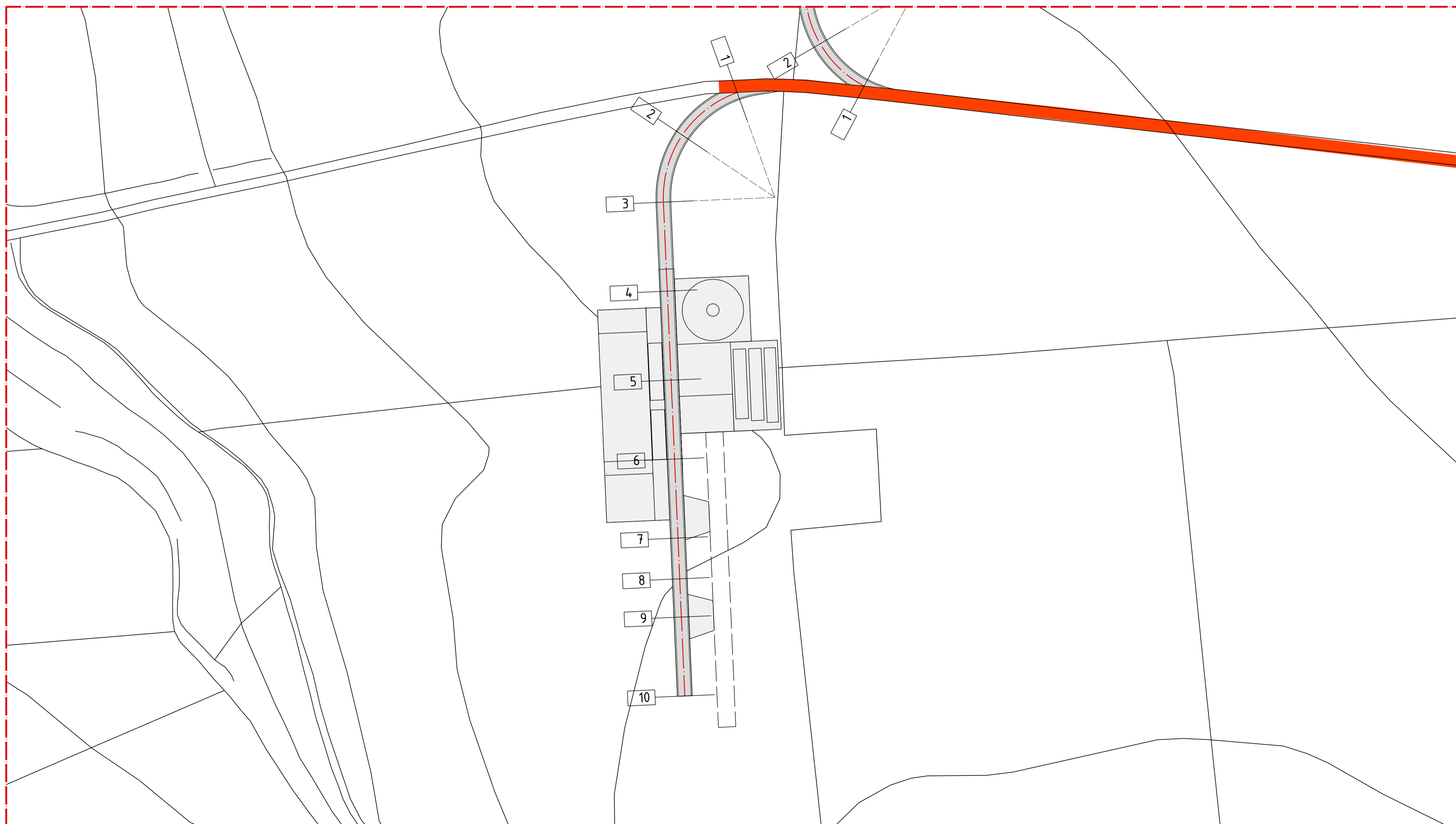
Planimetria WTG-D Scala 1:1.000
