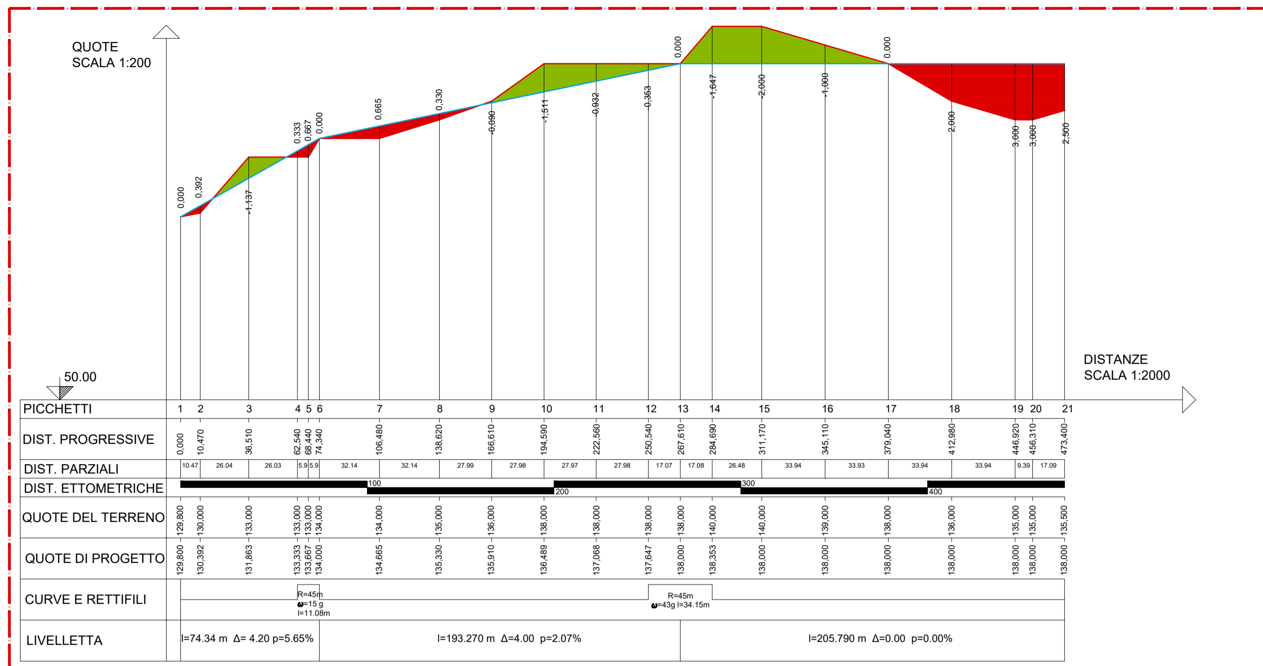
Profilo altimetrico WTG-L Scala 1:2.000
