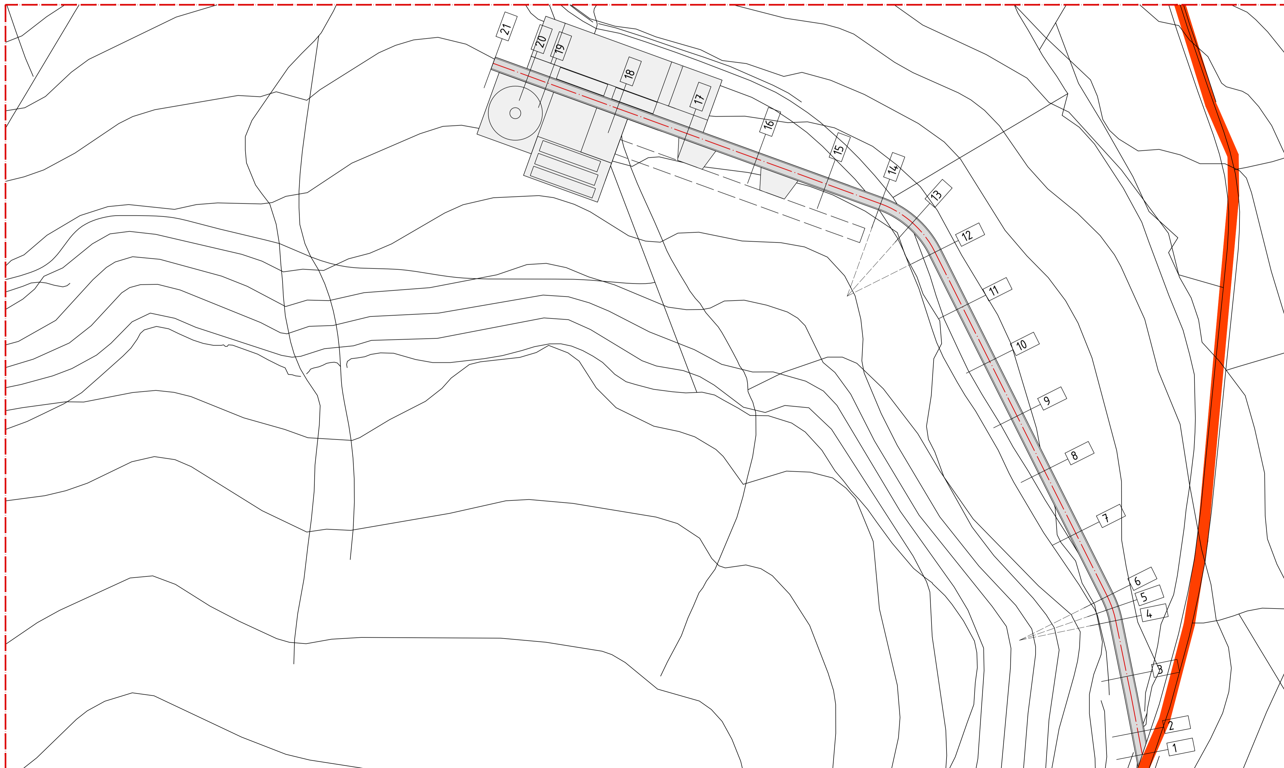
Planimetria WTG-L Scala 1:1.000
