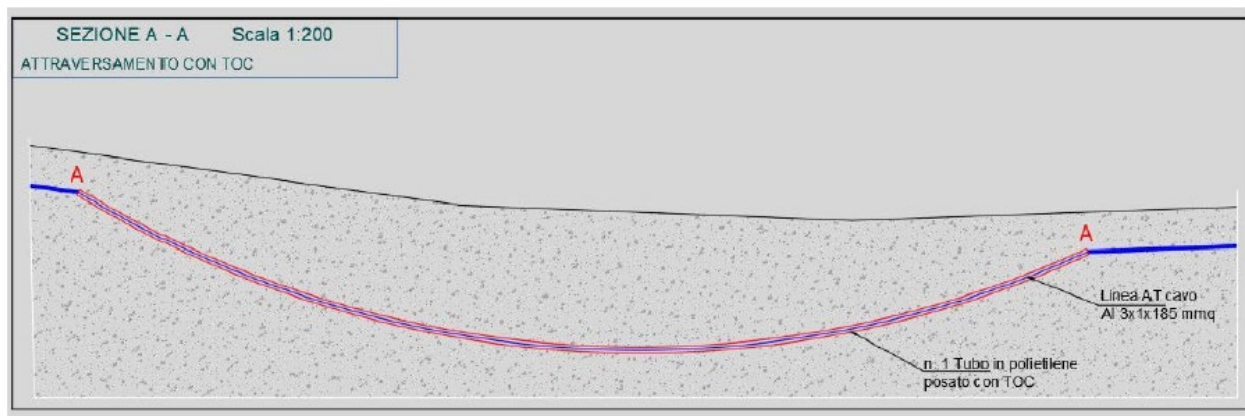
Figura 23 Attraversamento Reticolo Idrografico (TOC)
