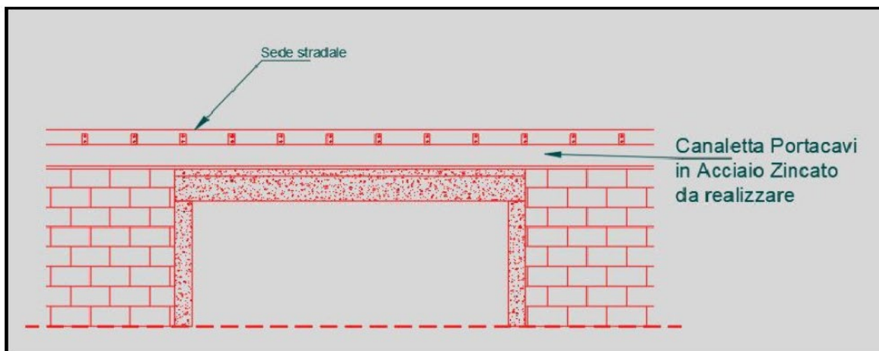
Figura 26 Attraversamento Reticolo Idrografico (Staffaggio a ponte)
