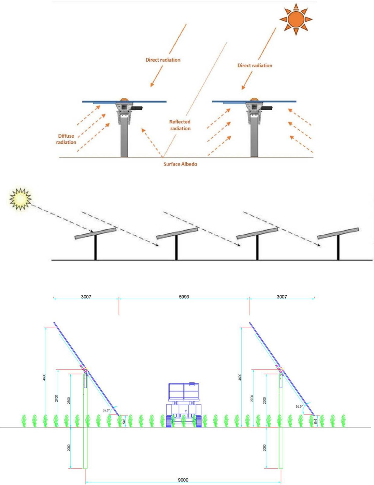
Figura 21 – schemi funzionali n dei pannelli
