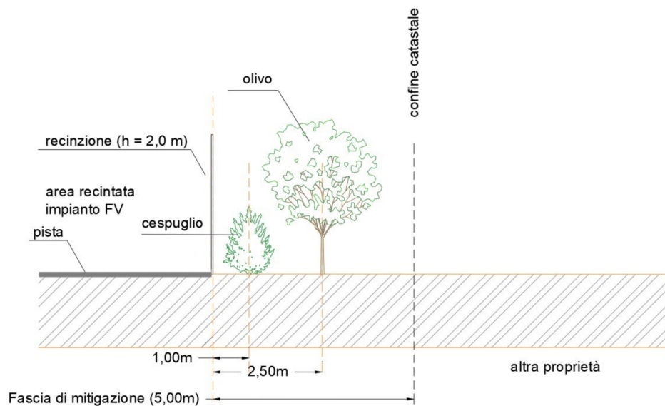
Figura 2.13. – Stralcio di sezione dell'area perimetrale dell'impianto.
