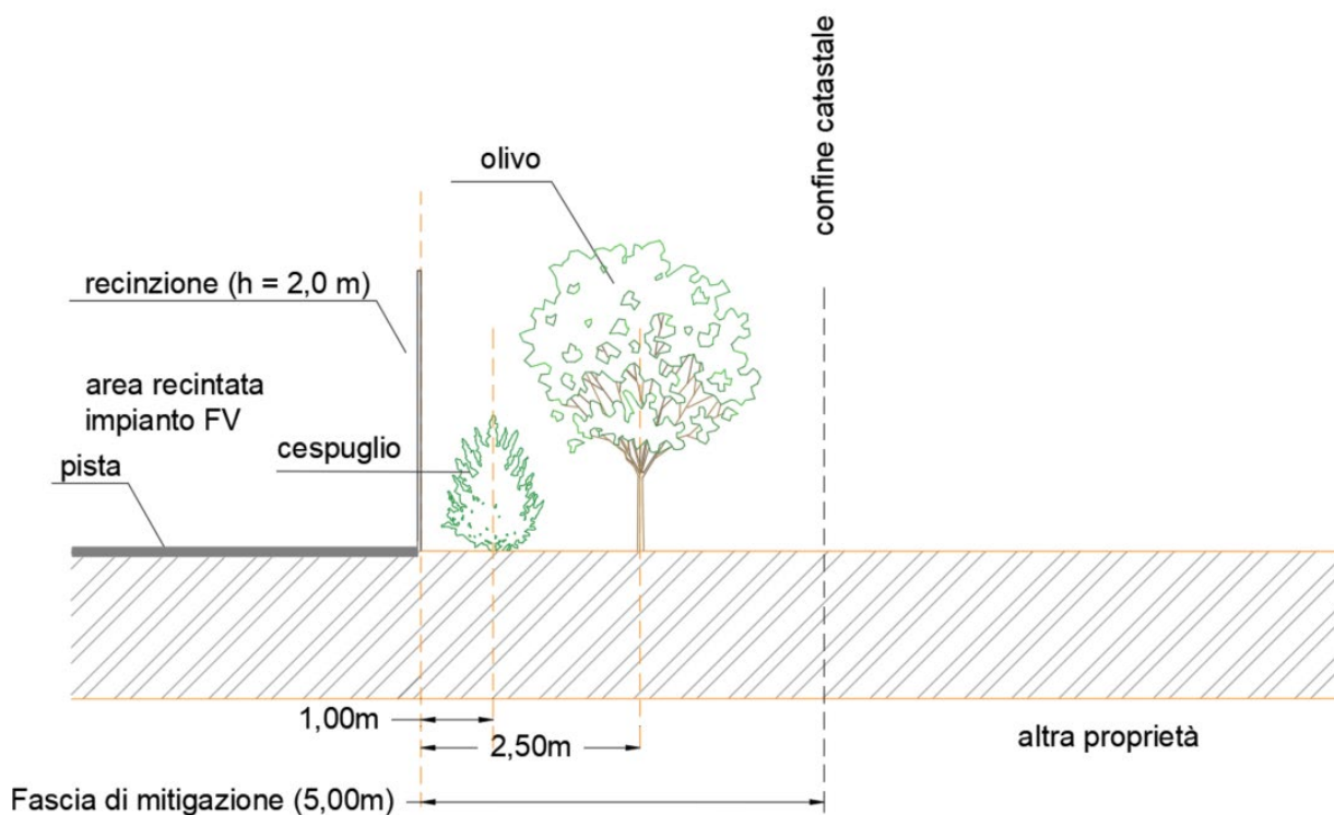
Figure 12.4. – Stralci di sezione dell'area perimetrale dell'impianto.
