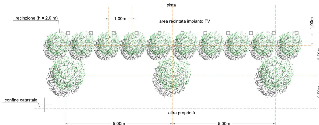
Figure 12.3. – Sezione polispecifica (planimetria di progetto).
