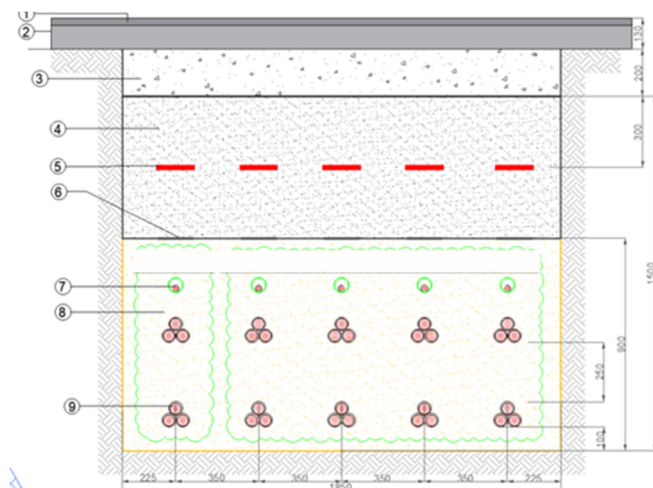
Figura 5. Sezione tipo sotto sede stradale
