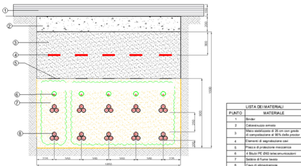
Figura 7. Sezione tipo in attraversamento su strada pubblica o in area Terna
