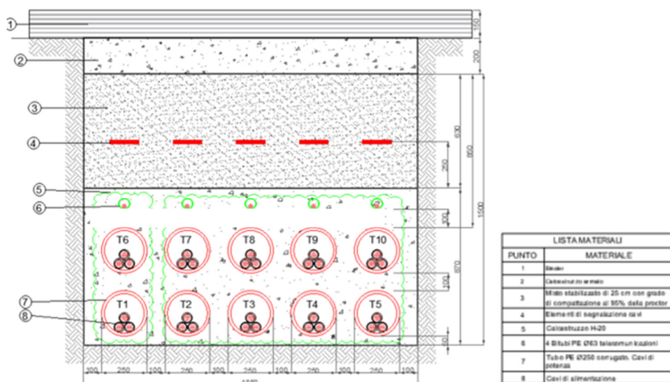
Figura 8. Sezione tipo canalizzazione dei tubi in cls in attraversamento su strada pubblica o in area Terna
