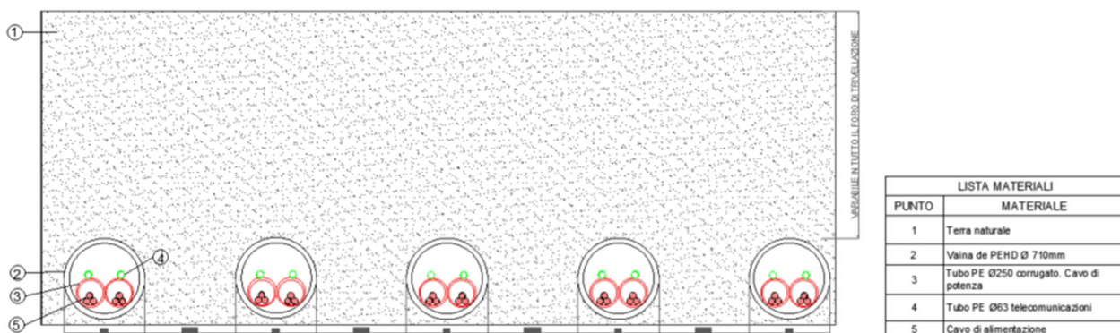
Figura 9. Sezione tipo in attraversamento in toc con tubo PHD Vaiana 710 mm e tubo 250 mm
