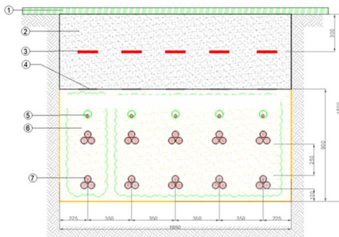
Figura 6. Sezione tipo in terreno vegetale
