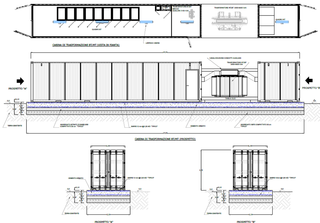
Fig.4 - Ingombri cabine di trasformazione AT/BT
