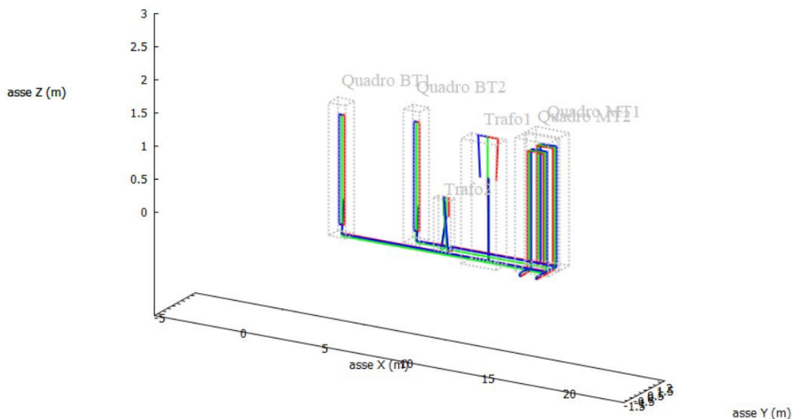
Fig.6 - Modello spaziale cablaggi nelle cabine di trasformazione AT/BT
