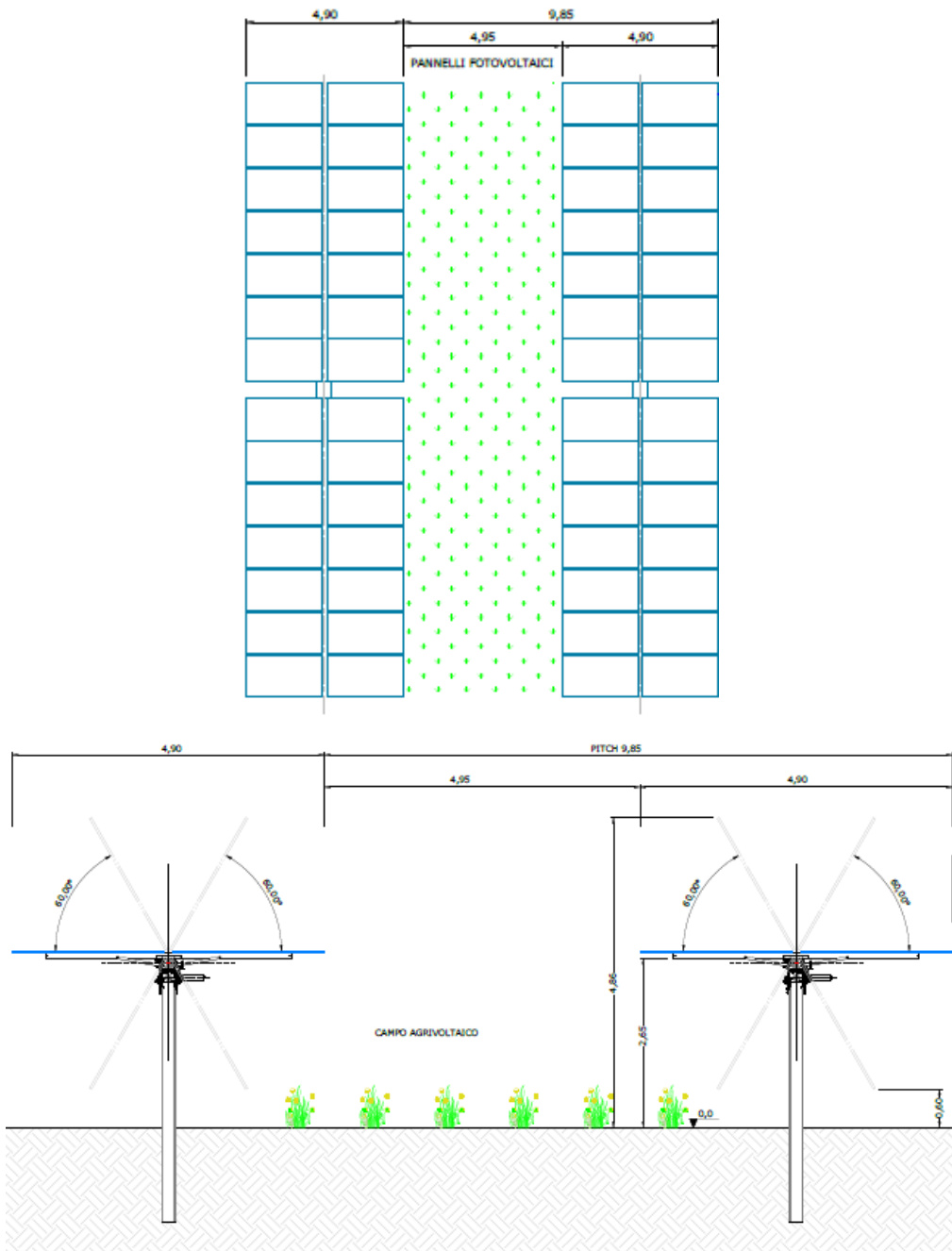
Fig. 2 – Piantumazione tra le file di tracker
