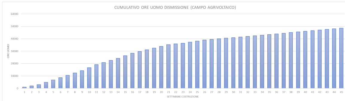
Fig. 7 – Istogramma n° addetti dismissione / cumulativo ore uomo costruzione (campo agrivoltaico)
