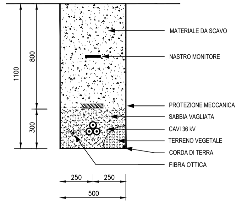
SEZIONE TIPO 1 Terne su TERRENO
