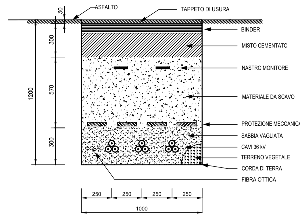
SEZIONE TIPO 3 Terne su STRADA
