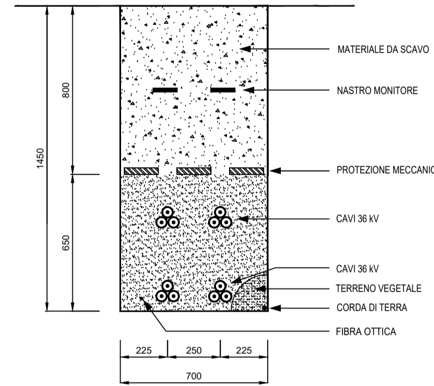
SEZIONE TIPO 4 Terne su TERRENO
