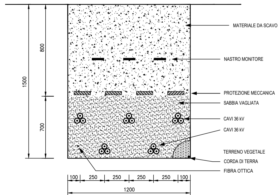
SEZIONE TIPO 5 Terne su TERRENO
