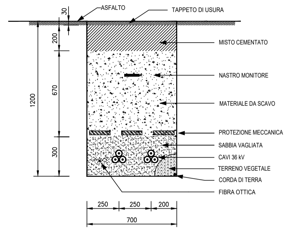
SEZIONE TIPO 2 Terne su STRADA
