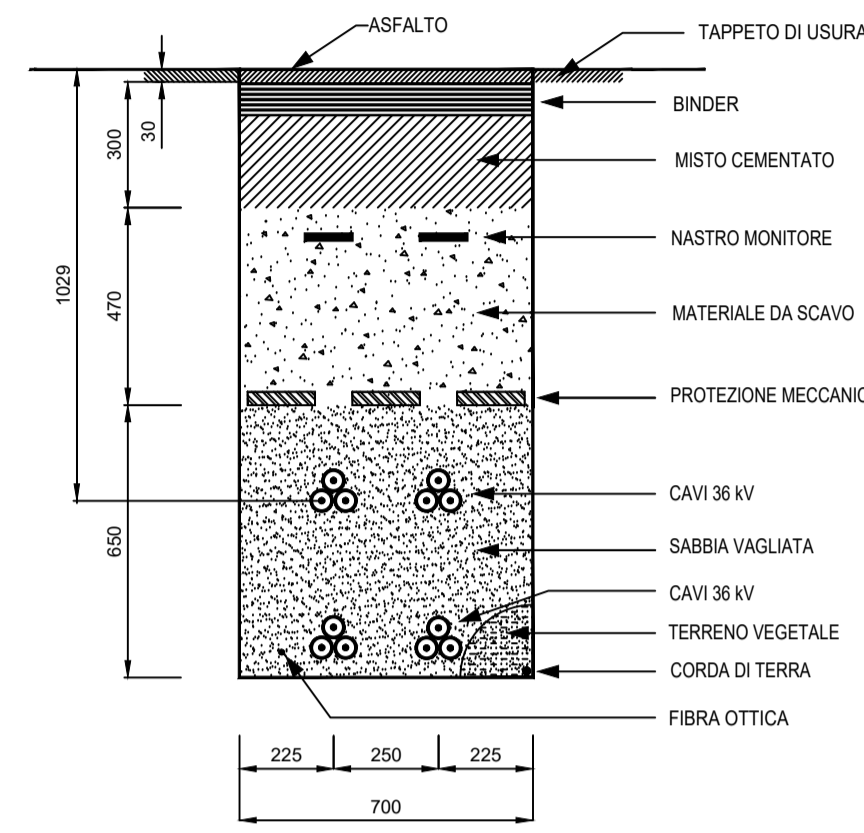
SEZIONE TIPO 4 Terne su STRADA
