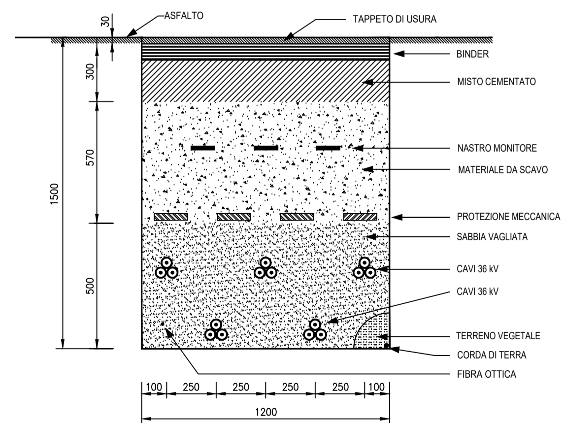
SEZIONE TIPO 5 Terne su STRADA
