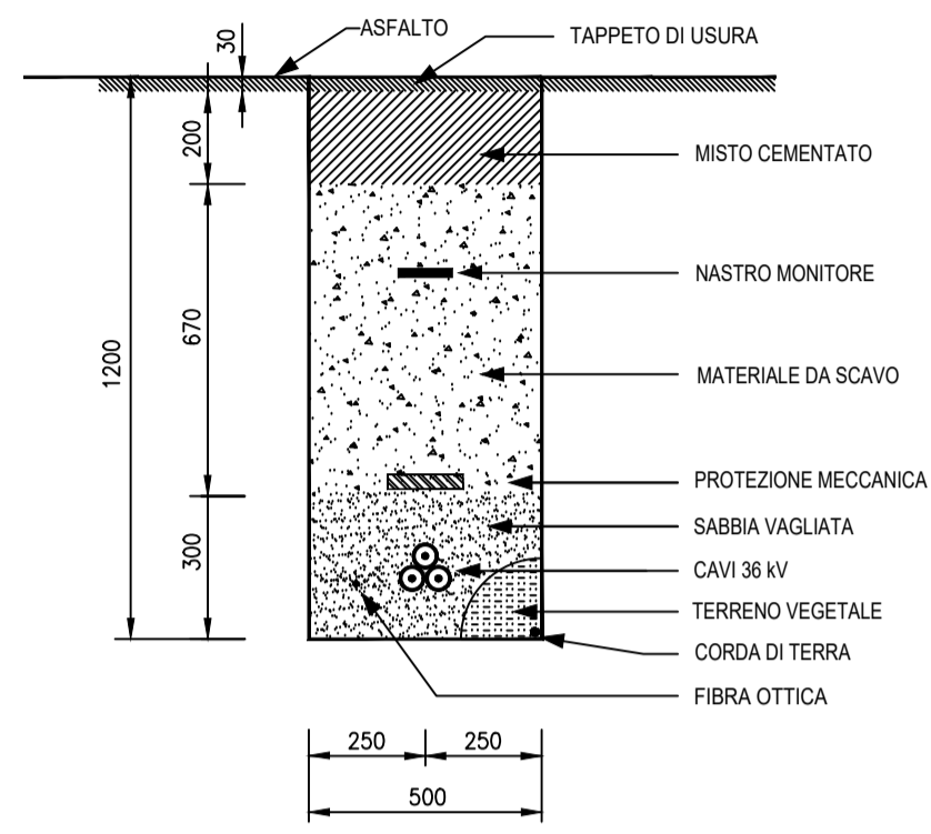
SEZIONE TIPO 1 Terne su STRADA
