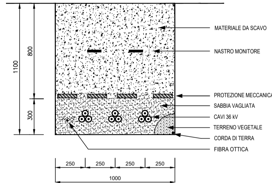
SEZIONE TIPO 3 Terne su TERRENO
