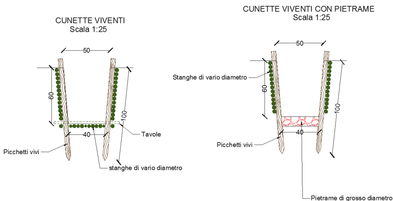
Figura 24 – Sezioni tipo di cunette viventi
