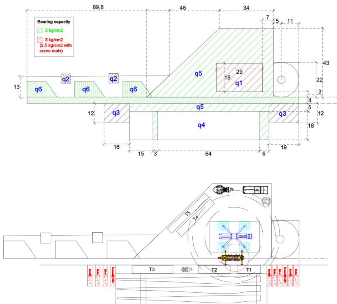
Figura 14 - Piazzola aerogeneratore durante la fase di montaggio
