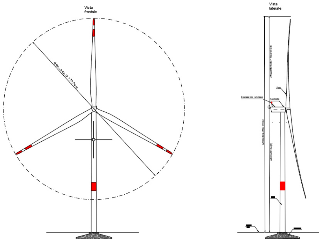
Figura 31 - Pianta e prospetti aerogeneratore m
